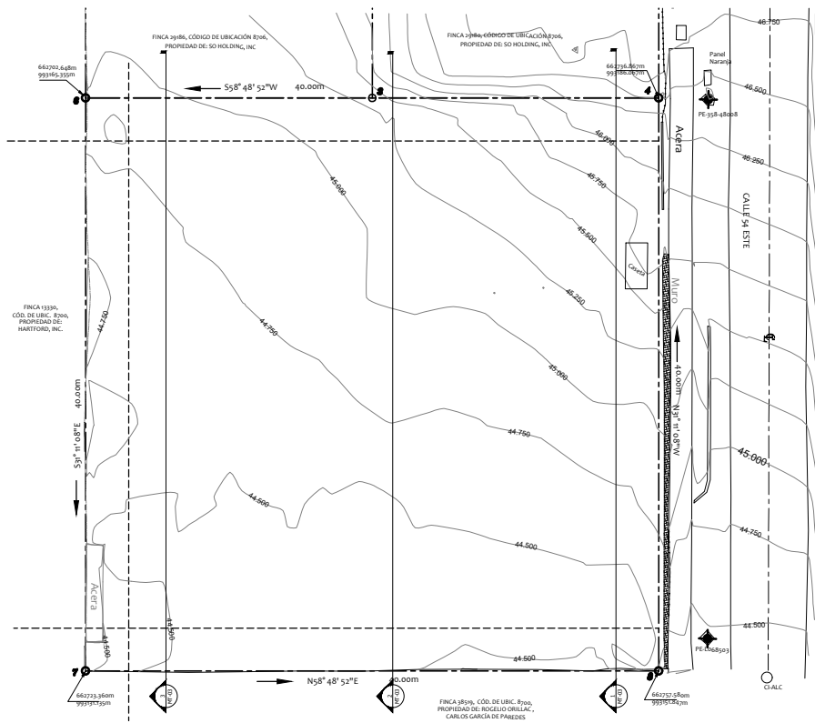
PLANTA GENERAL DE TOPOGRAFÍA EXISTENTE
