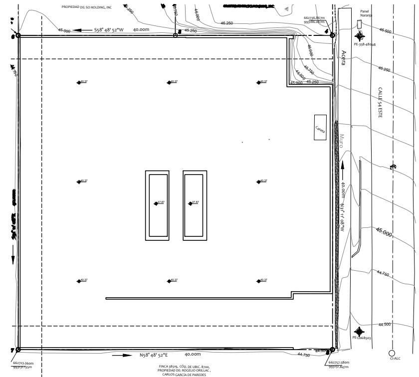
PLANTA GENERAL DE CURVAS DE NIVEL MODIFICADAS
