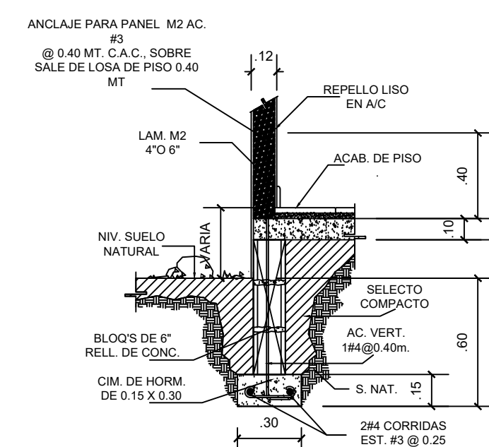
CIMIENTO TIPO ESCALA 1:20 C A
