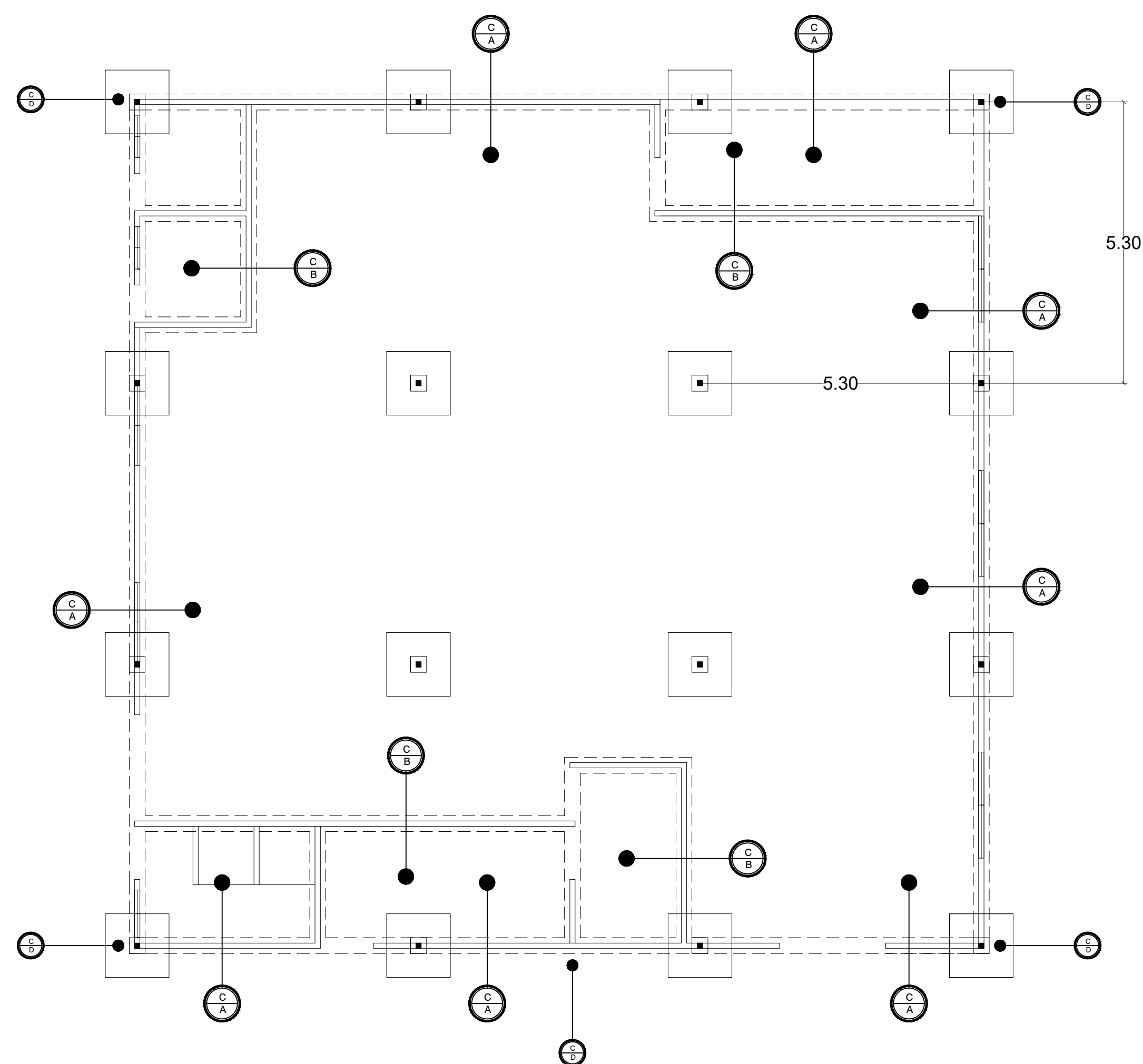
PLANTA DE CIMIENTOS ESC. 1:75
