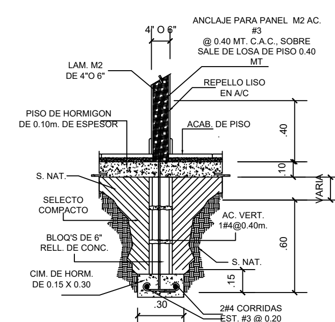
CIMIENTO TIPO ESCALA 1:20 C B
