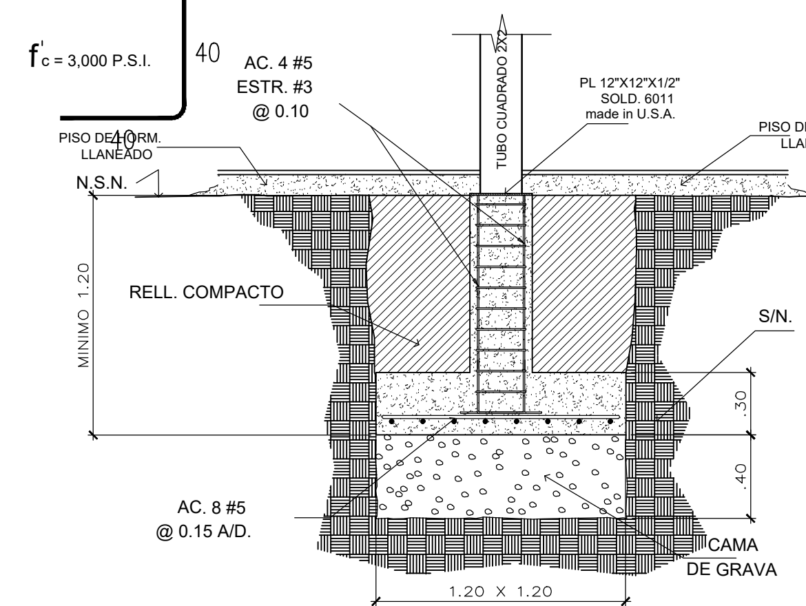
CIMIENTO TIPO C D ESCALA 1:20
