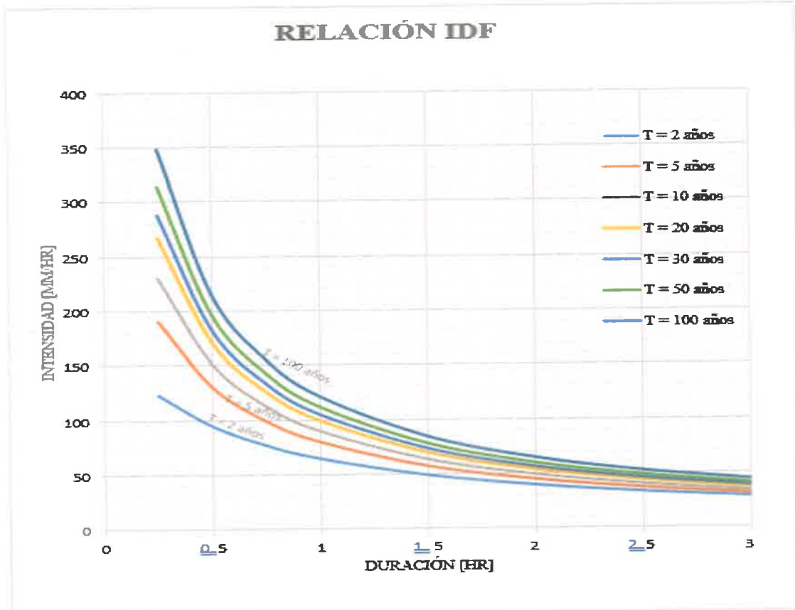
Gráfica 4. 12: 144 - Relación Intensidad Duración Frecuencia
