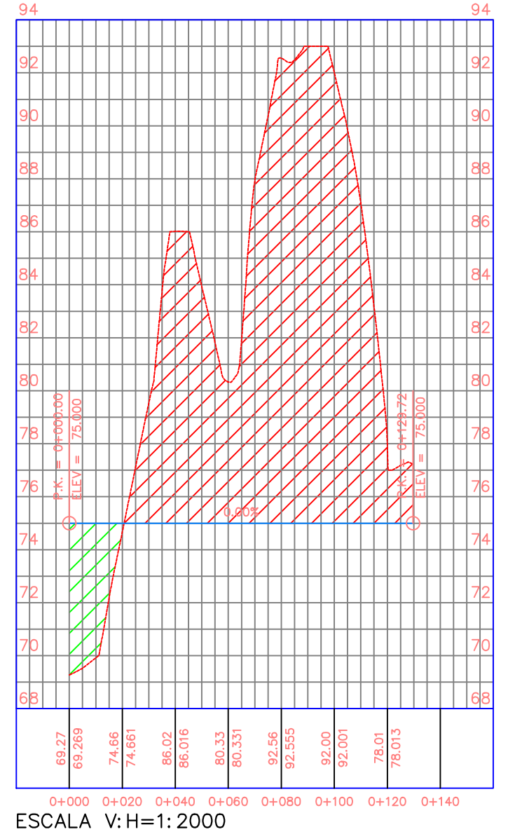
Alineamiento T2 PROFILE
