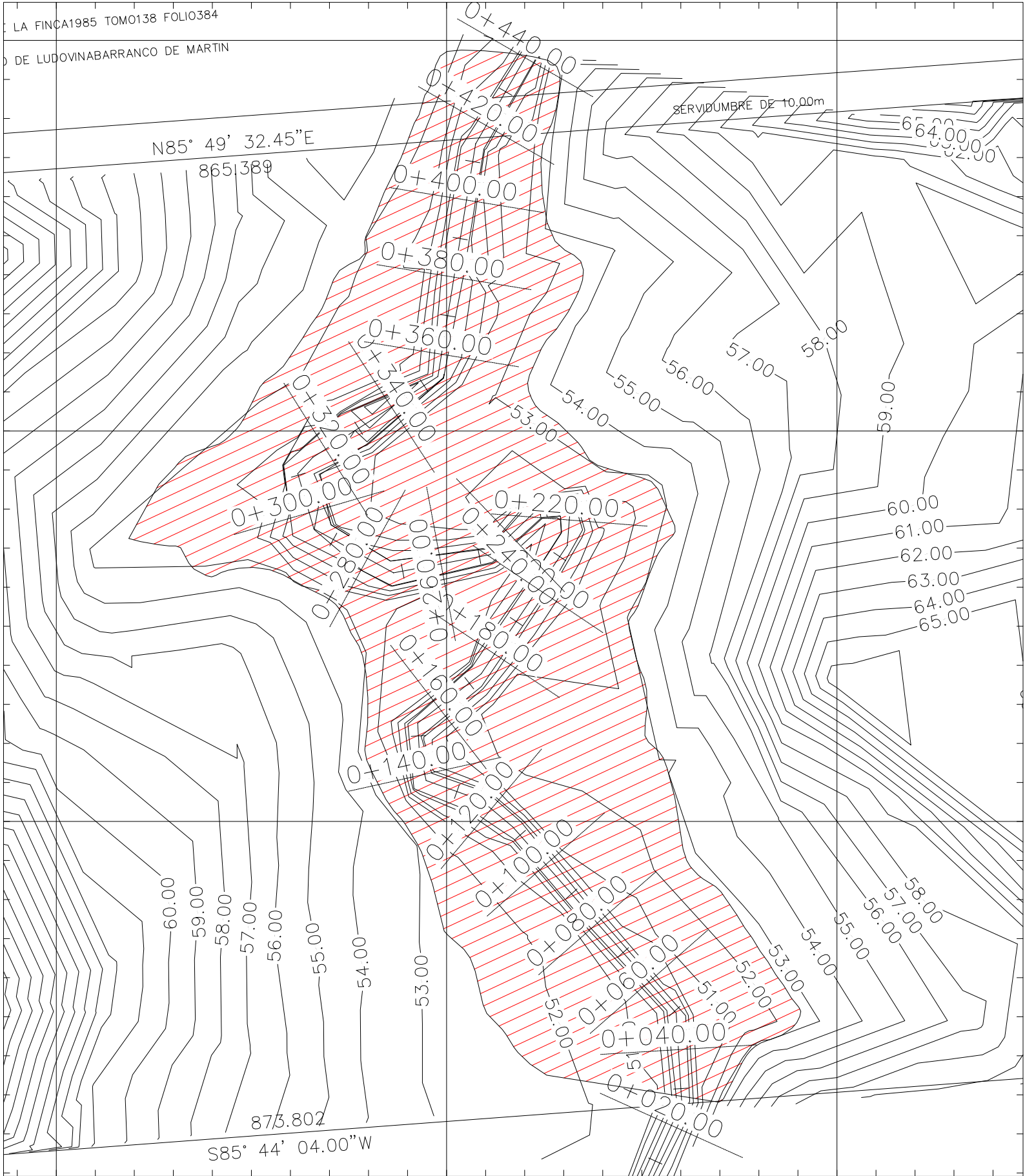
PLANICIE DE INUNDACIÓN 1:50 AÑOS ESC. 1:1250
