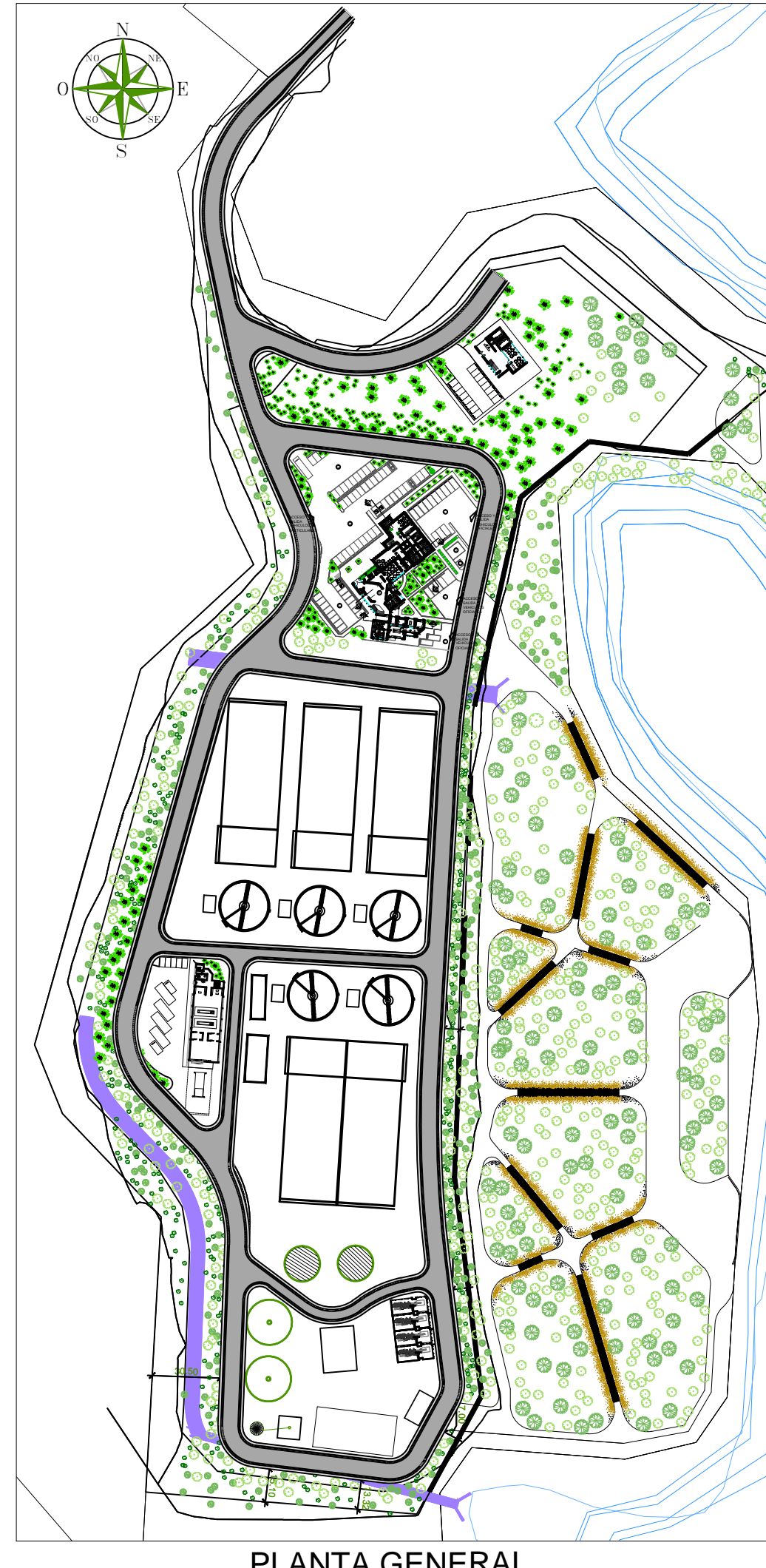
PLANTA GENERAL
