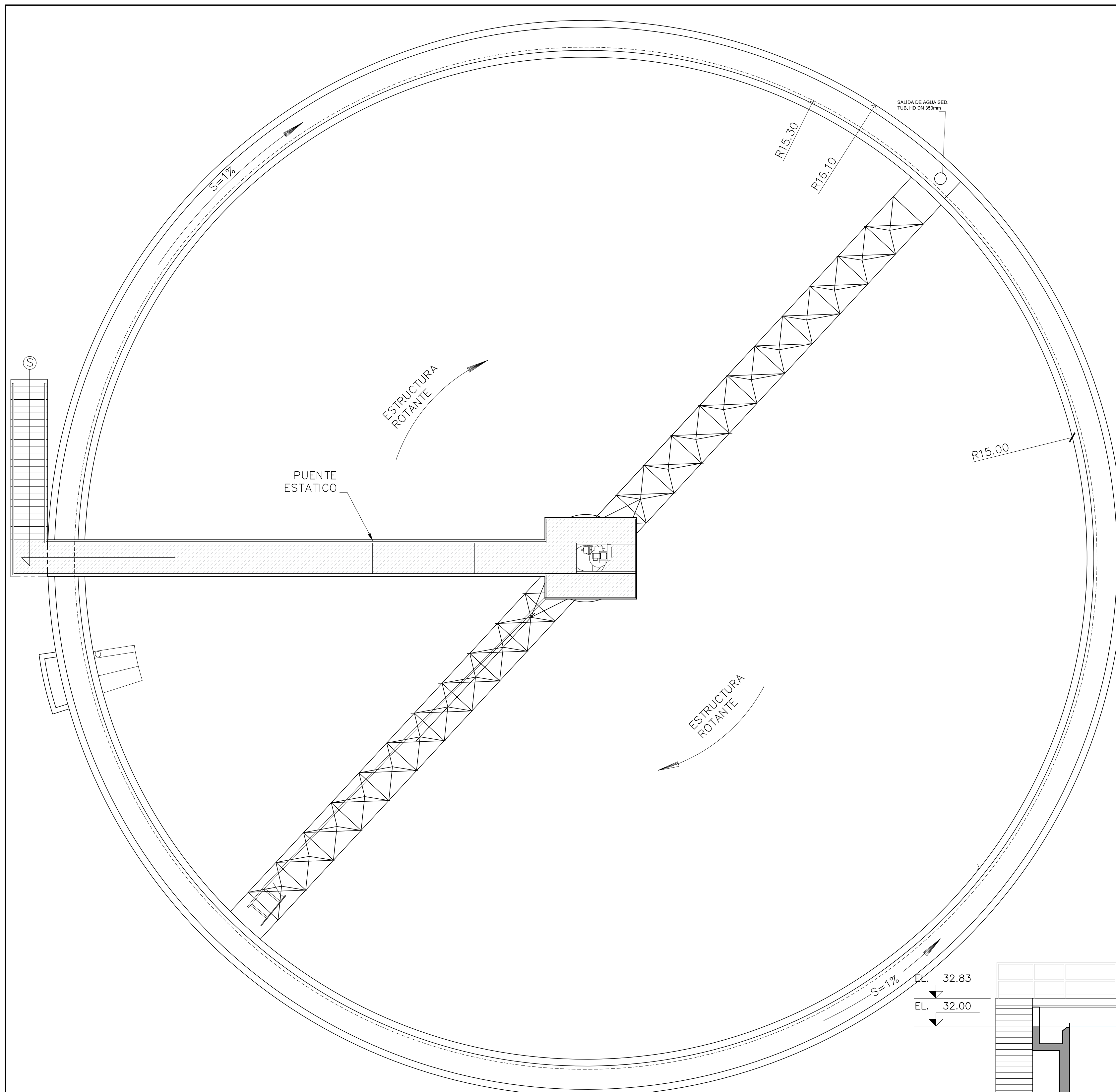
A PLANTA – SEDIMENTADOR ESCALA: 1:75
