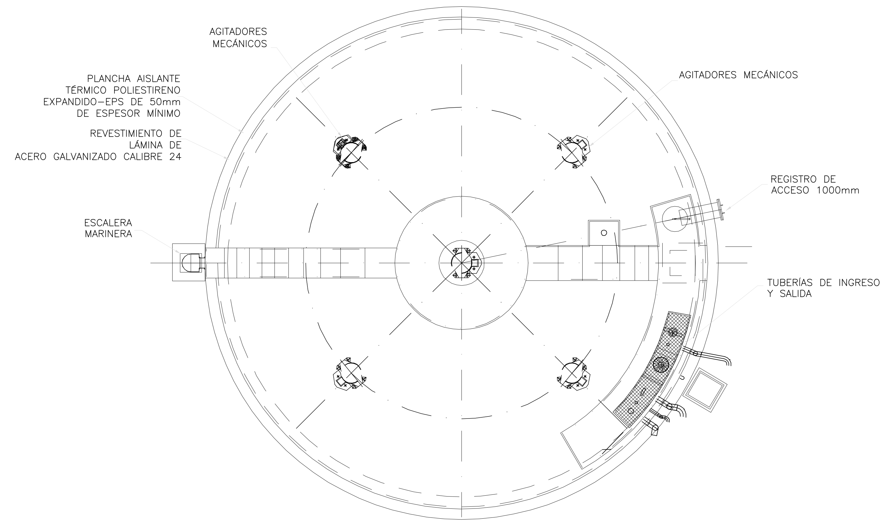
DIGESTOR PRIMARIO PLANTA
