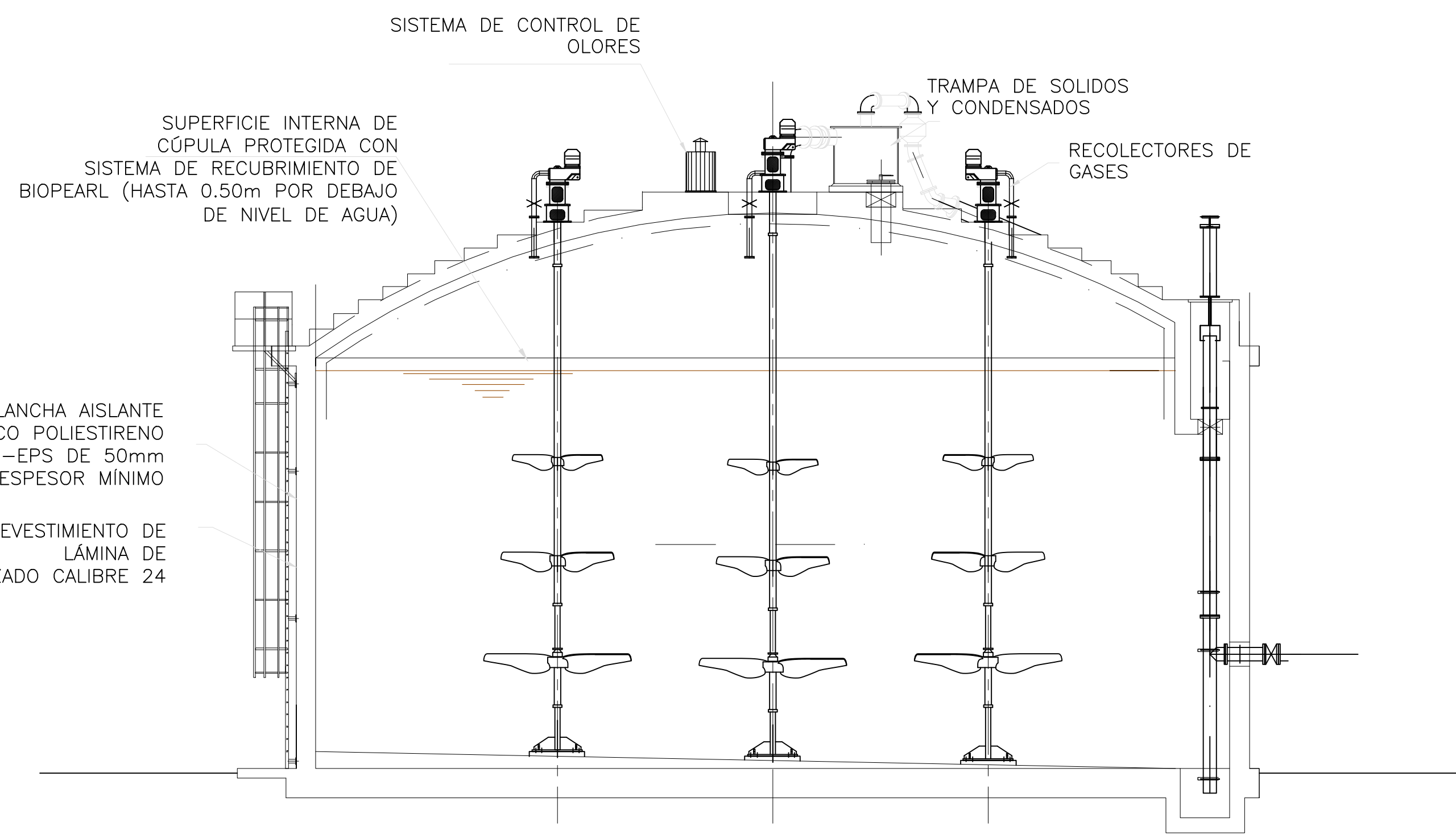
DIGESTOR PRIMARIO SECCIÓN A-A
