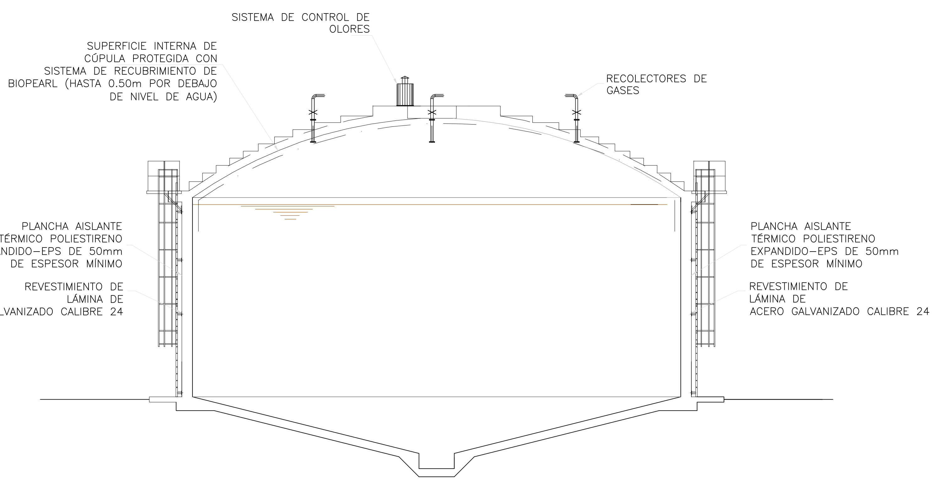
DIGESTOR SECUNDARIO SECCIÓN A-A
