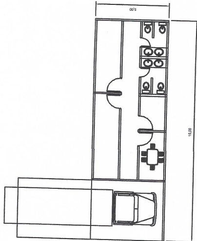
PLANTA DE OFICINAS
