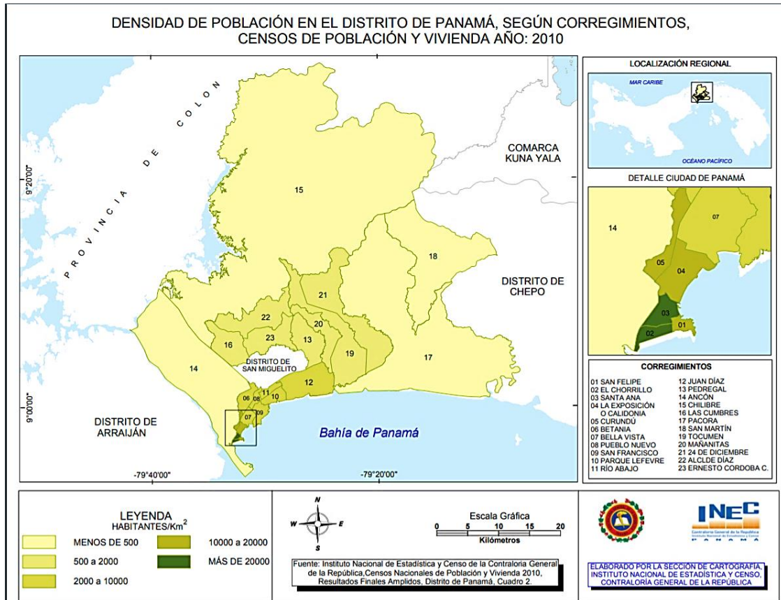
Figura N° 8.5 – Mapa de densidad Poblacional.
