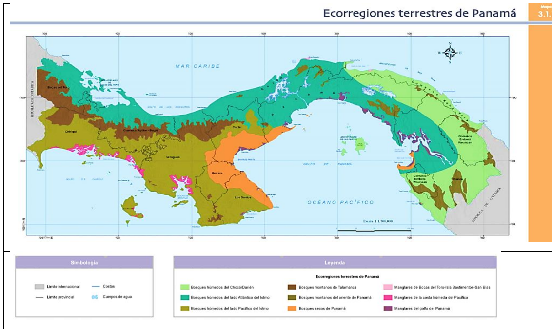
Figura No 7.1. Mapa de ecorregiones. El proyecto se ubica en la Ecorregión del Bosques Húmedos del Atlántico del Istmo. Fuente: Atlas Ambiental 2010.
