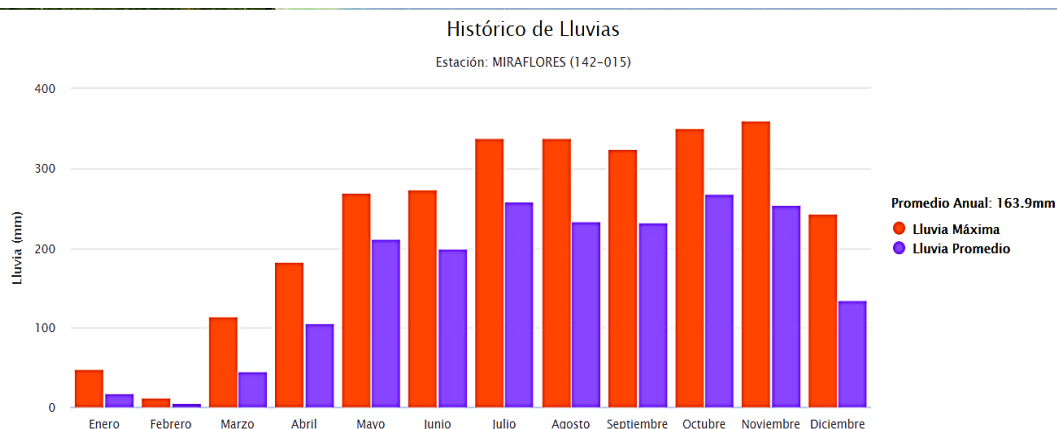
Figura 6.15: Gráfico de Datos Históricos Estación Miraflores (Lat 9°00'51" y Lon -79°36'36", 20 msnm)
