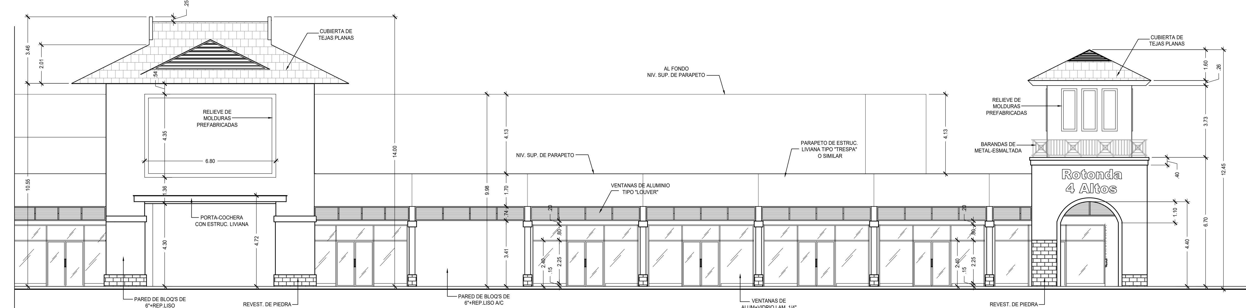
ELEVACION FRONTAL (PARTE 2)
