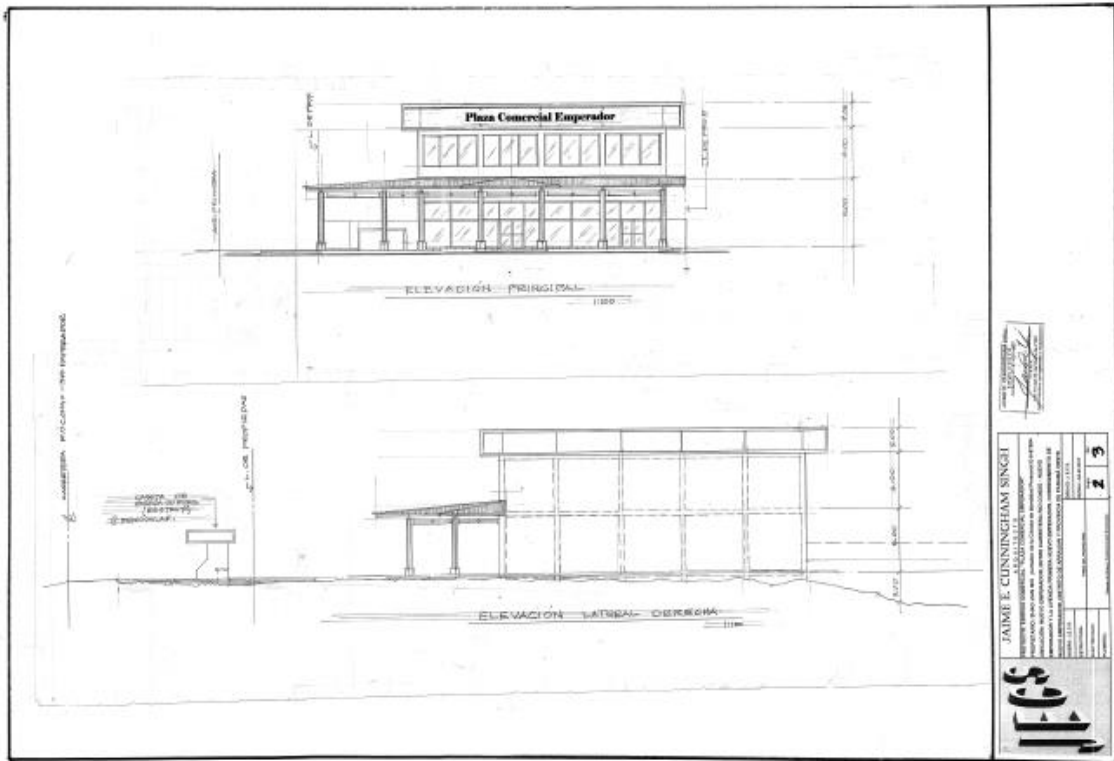
Figura N°4: Elevación Principal Y Lateral Derecha
