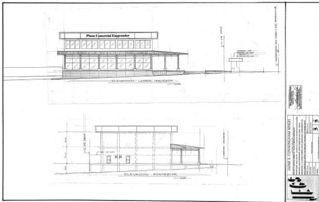
Figura Nº5: Elevación Lateral Izquierda Y Posterior
