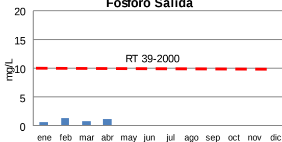
Fósforo Salida
