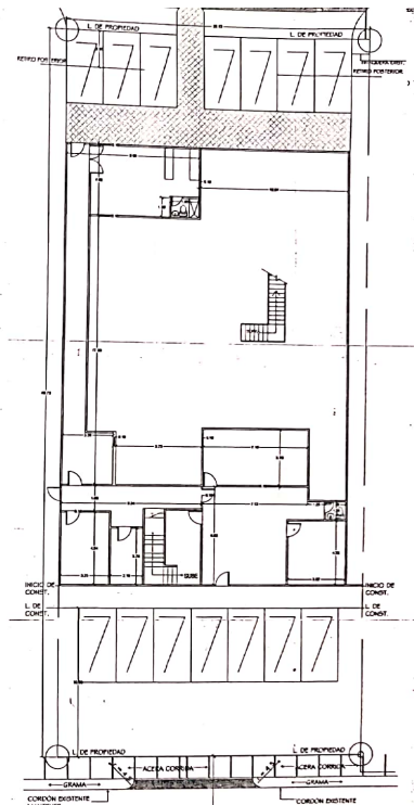
PLANTA ARQUITECTONICA # LOCALIZACION ESC. 1/200
