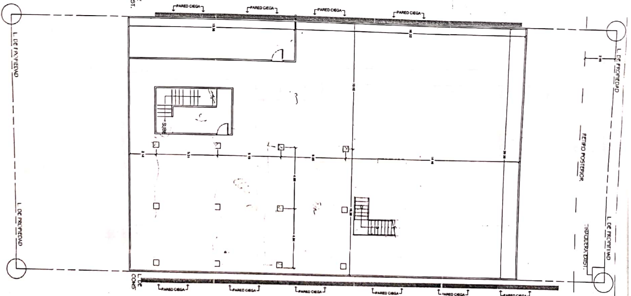
PLANTA ALTA NIVEL 100 Esc. 1/100
