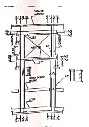
REFUERZO ALREDEDOR DE VENTANA ESC. 1/200
