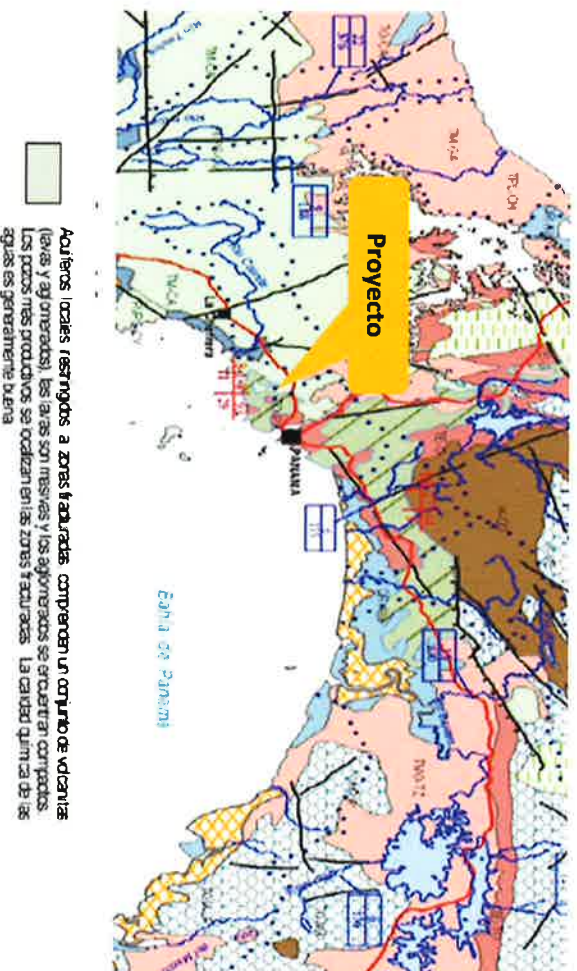
Imagen N°5: Extracto de Mapa Geológico de Panamá
