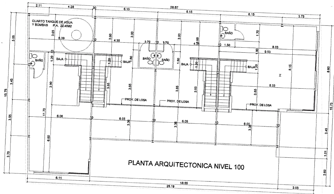
Figura 5. Planta arquitectónica baja – Nivel 100 (Fuente: Planos del proyecto)
