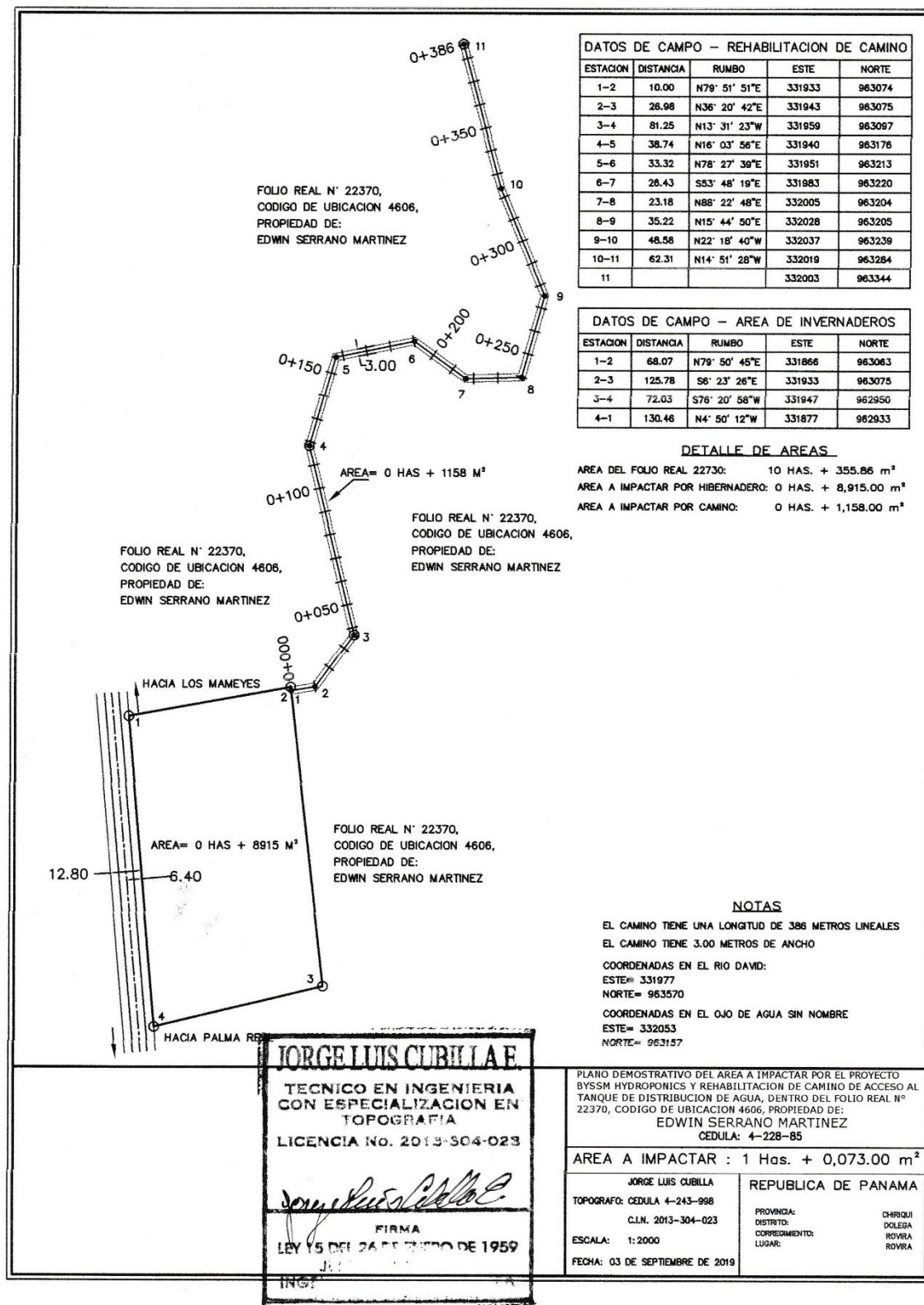
Figura 2. Plano del proyecto Fuente: El promotor
