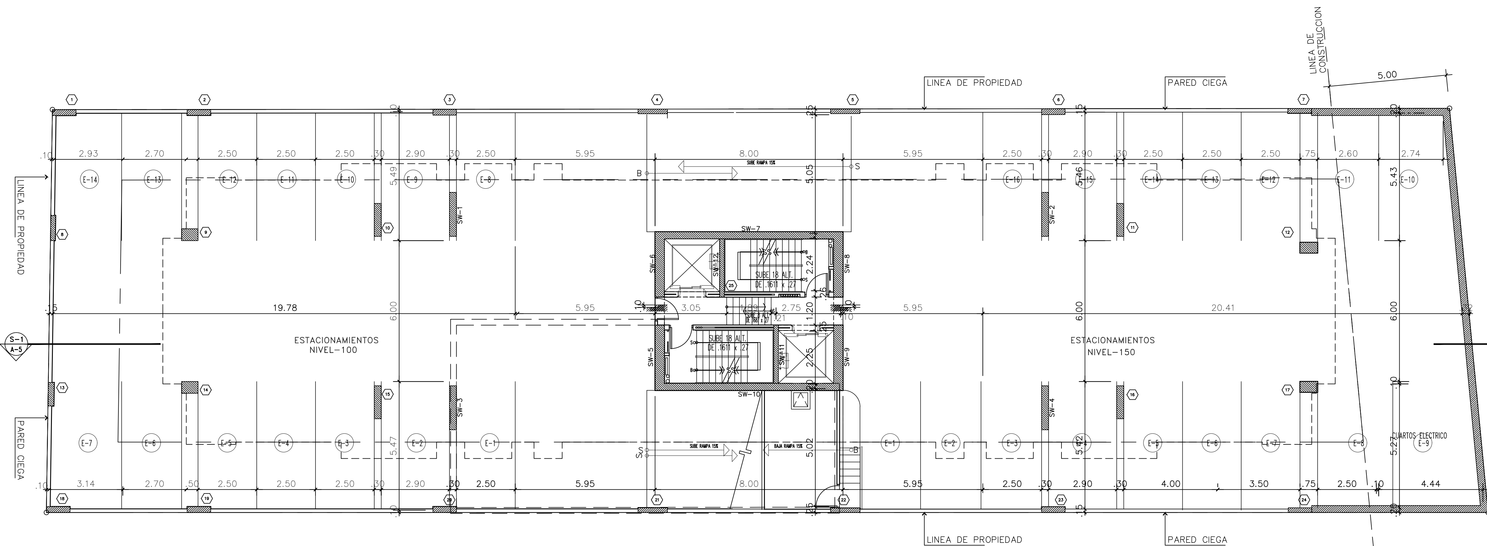
PLANTA ARQUITECTONICA NIVEL -100 Y -150
