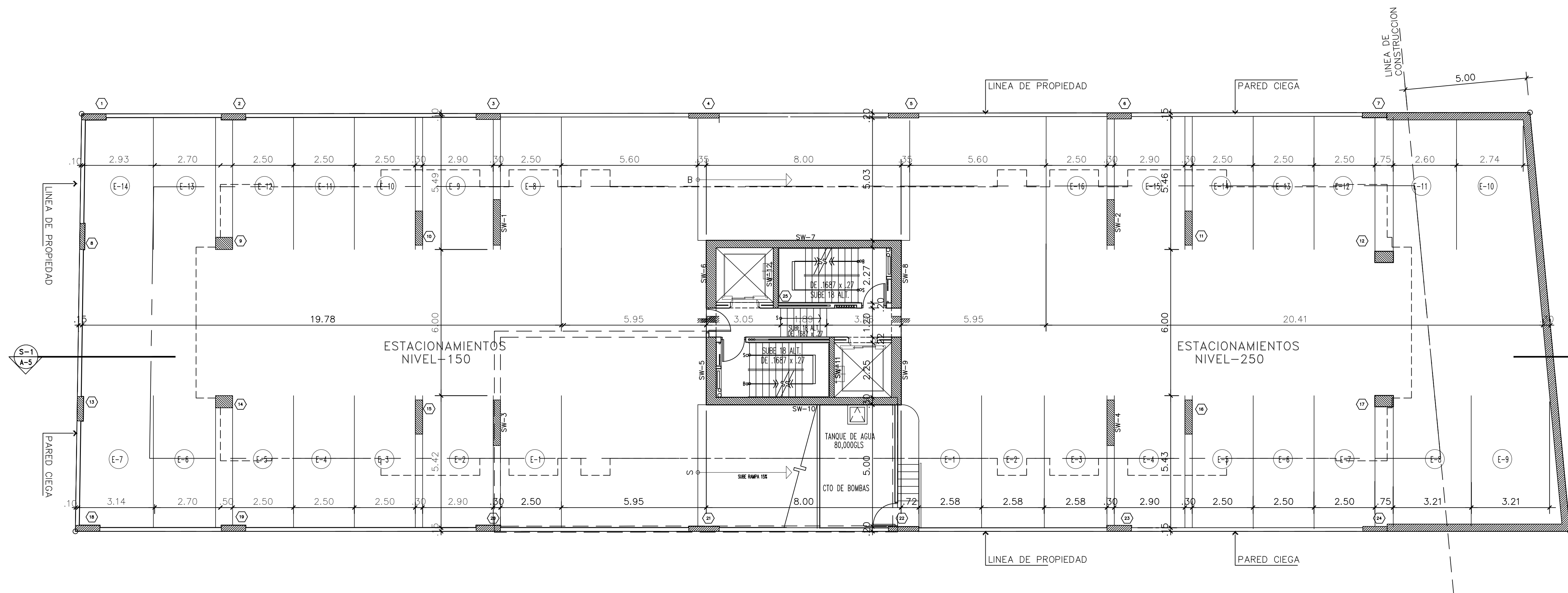
PLANTA ARQUITECTONICA NIVEL -150 Y -250
