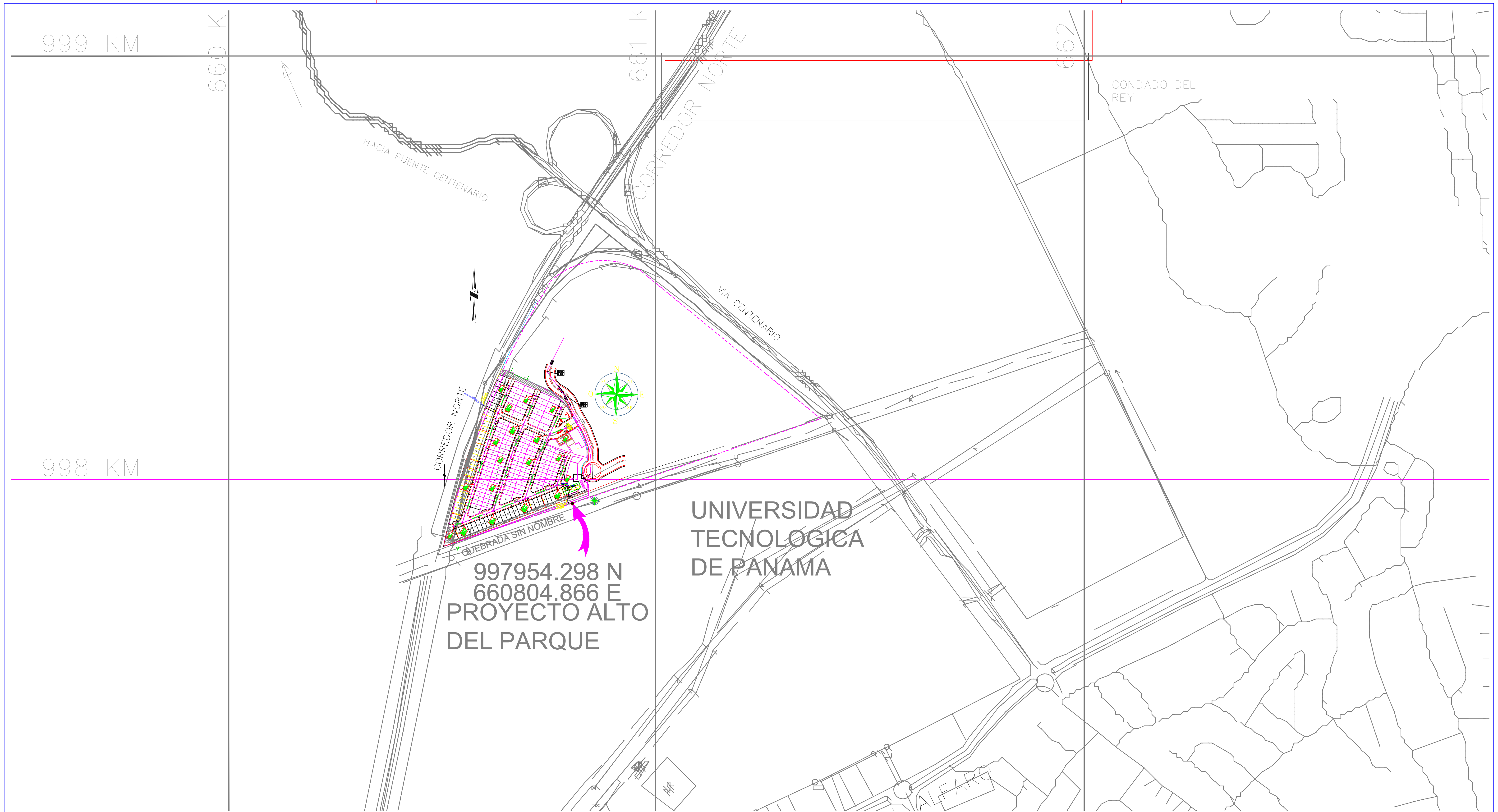
LOCALIZACION REGIONAL Y TOPOGRAFICA DE PLANTA DE TRATAMIENTO DE URBANIZACION ALTOS DEL PARQUE
