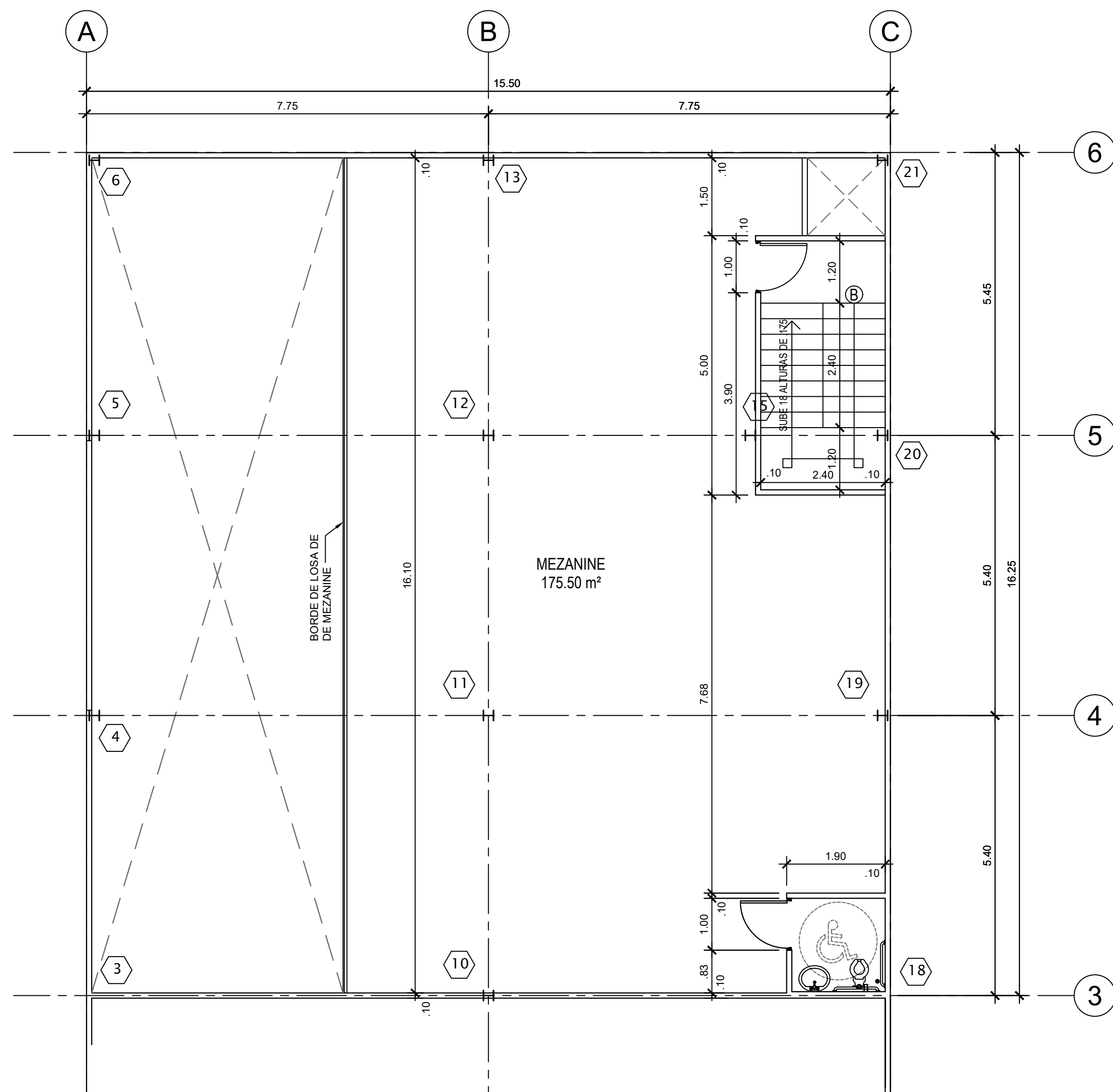
PLANTA AMPLIADA DE MEZANINE ESC.: 1:75
