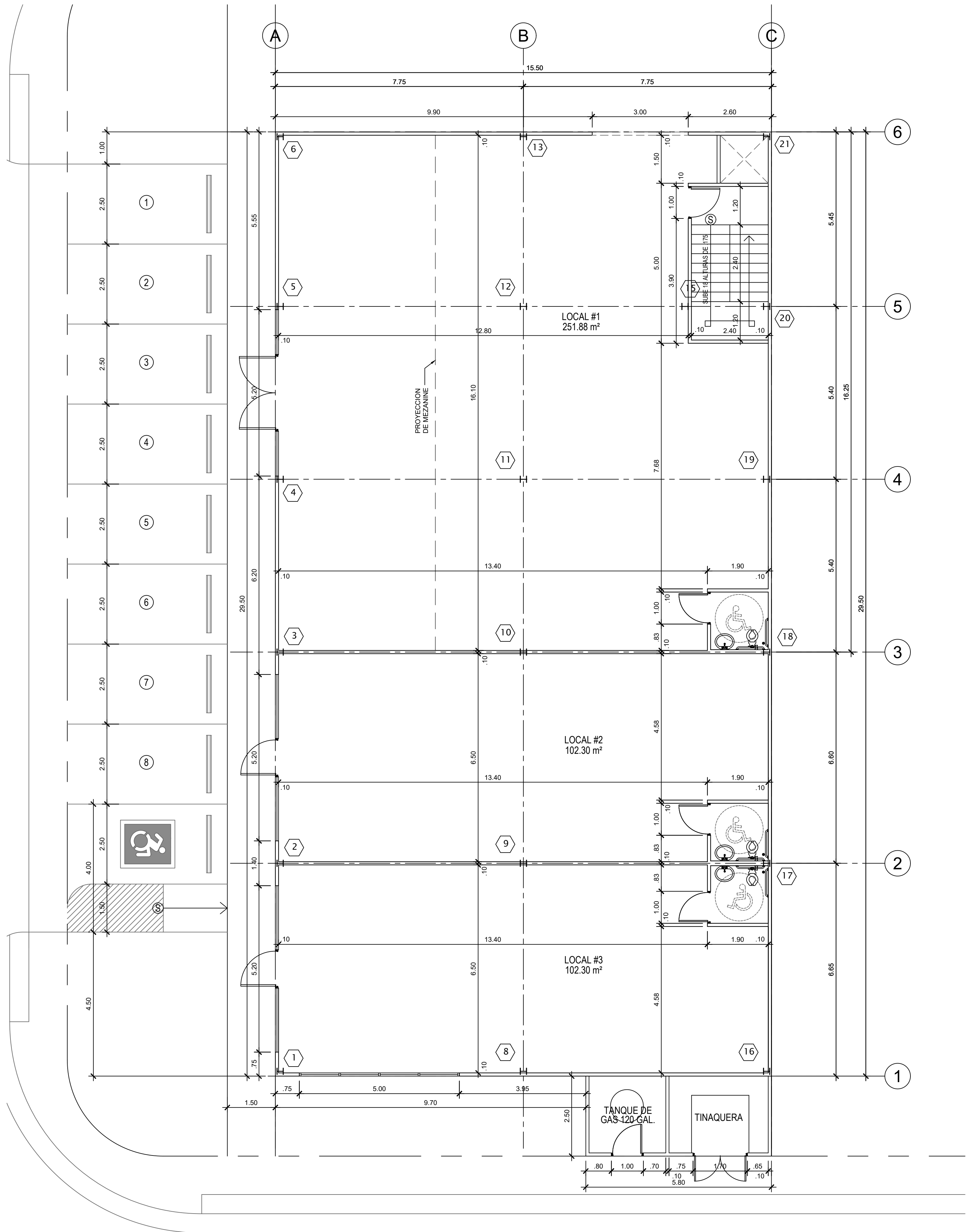
PLANTA BAJA ARQUITECTONICA AMPLIADA ESC.: 1:75
