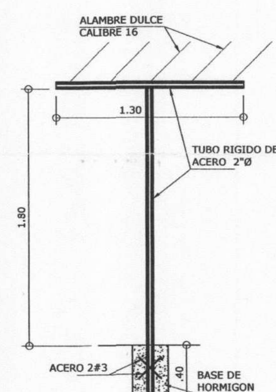
DET. DE TENEDERO ESC. 1:25
