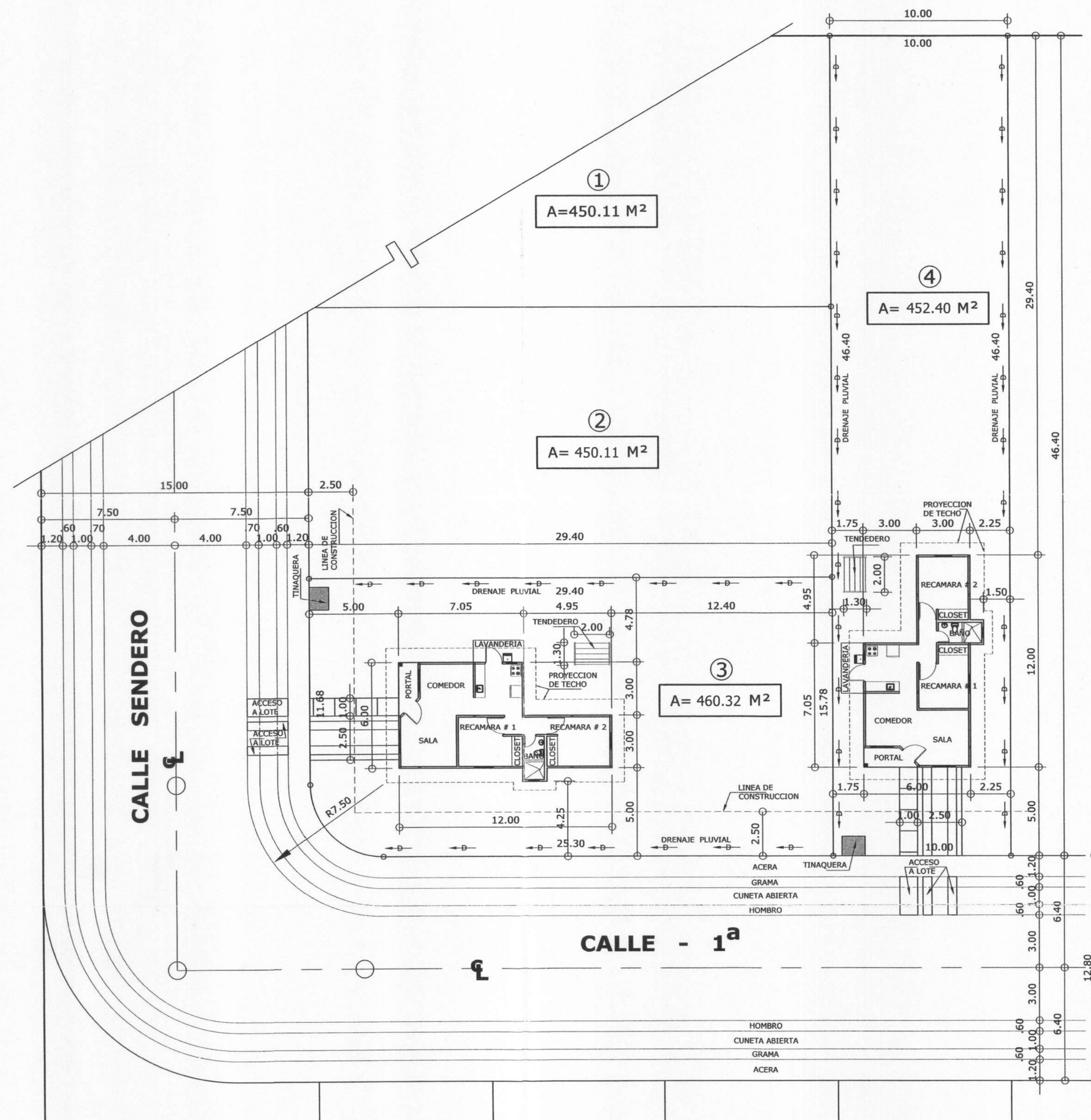
LOCALIZACIÓN DE VIVIENDA EN EL LOTE TÍPICO ESC. 1:150
