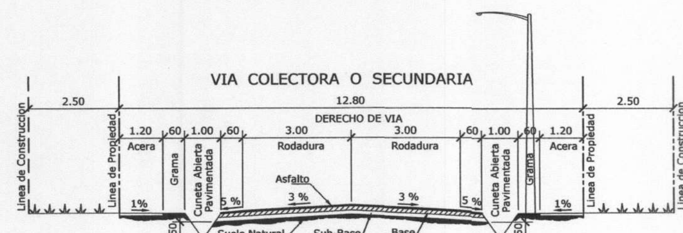
SECCION DE CALLE SECUNDARIA DE 12.80 m ESC. 1: 100
