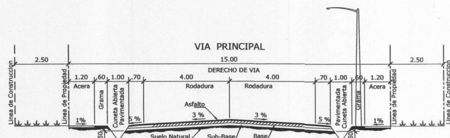
SECCION DE CALLE PRINCIPAL DE 15.00 m ESC. 1: 100
