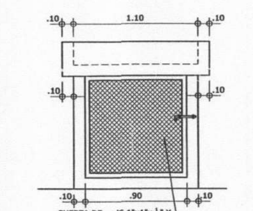
DET. TINAQUERA DE BLOQUES ESC. 1:33 1/3
