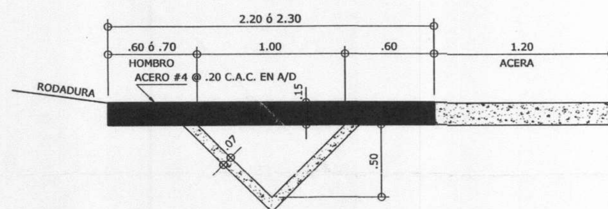
DET. DE ACCESO A LOTES ESC. 1:25
