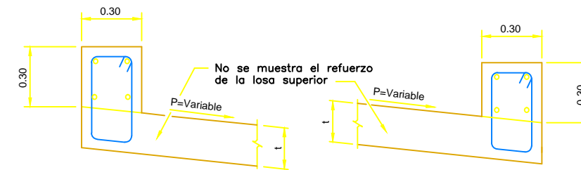
CABEZOTE SUPERIOR SIN ESCALA
