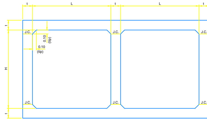
SECCIÓN TÍPICA DEL CAJÓN PLUVIAL SIN ESCALA
