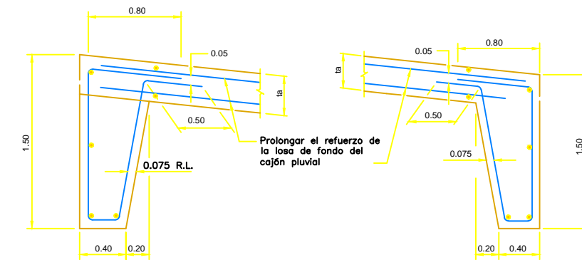
UÑA DE ENTRADA DE LA ALETA SIN ESCALA
