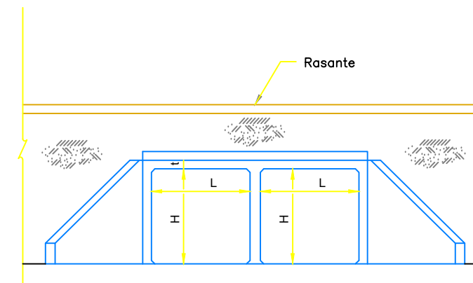
VISTA DE LA ENTRADA O DE LA SALIDA SIN ESCALA
