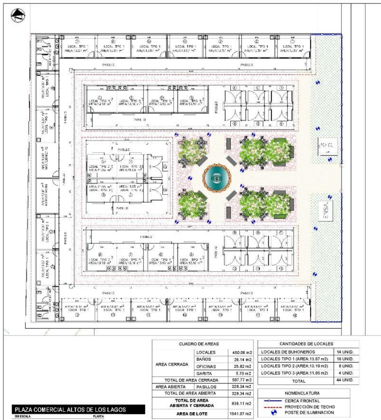
Figura 1: Arreglo general de la Plaza Comercial
