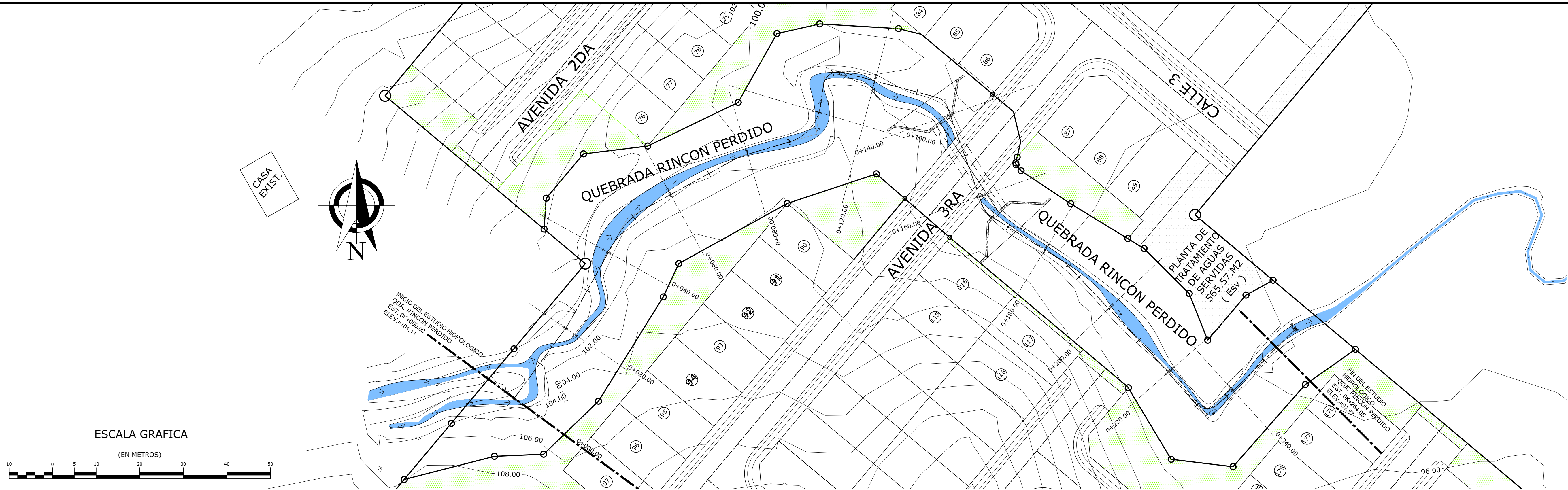
PLANO PERFIL DE QDA. RINCON PERDIDO ESC. 1 :500
