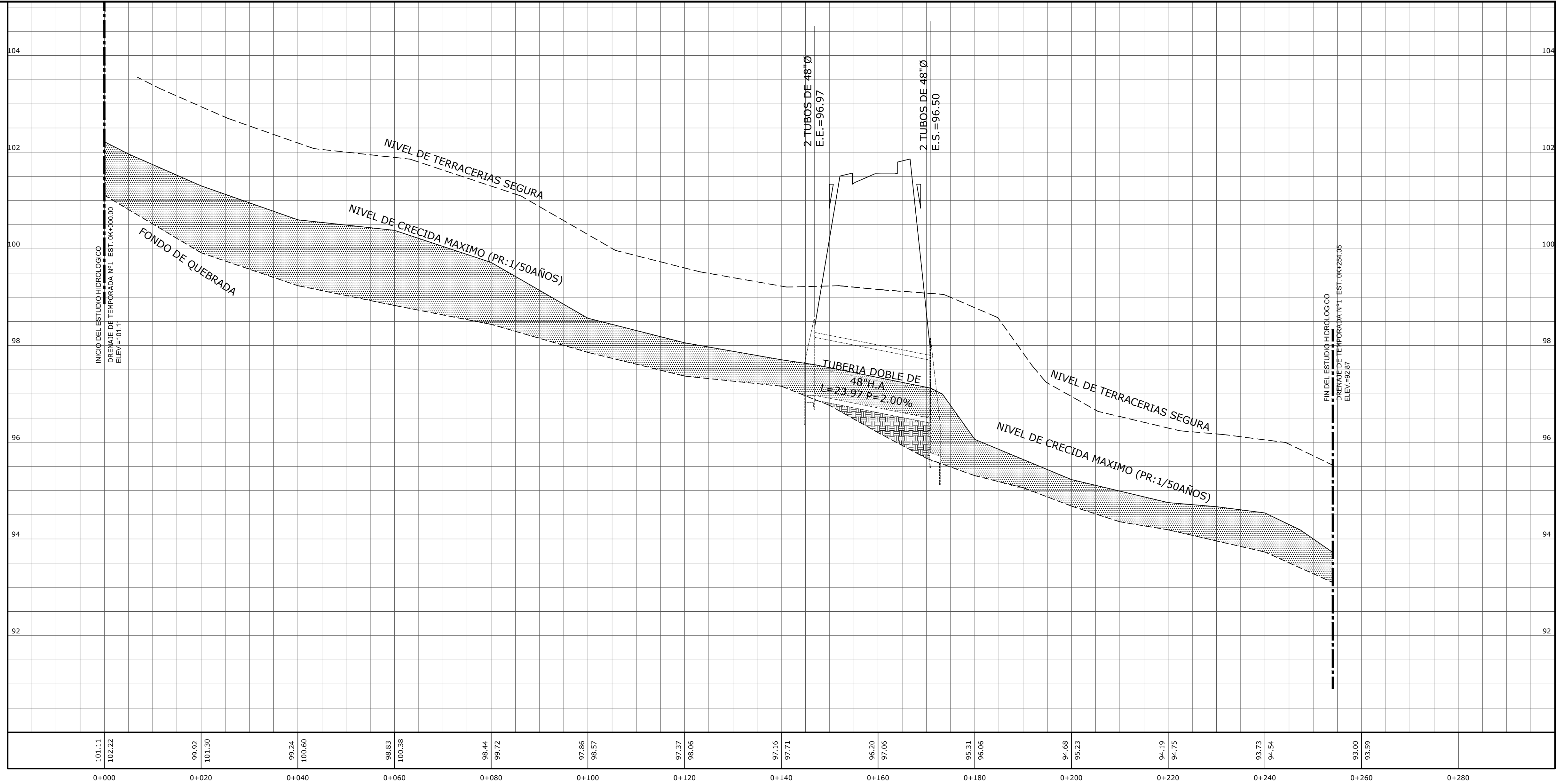
PLANO PERFIL DE QDA. RINCON PERDIDO ESC. 1 :500
