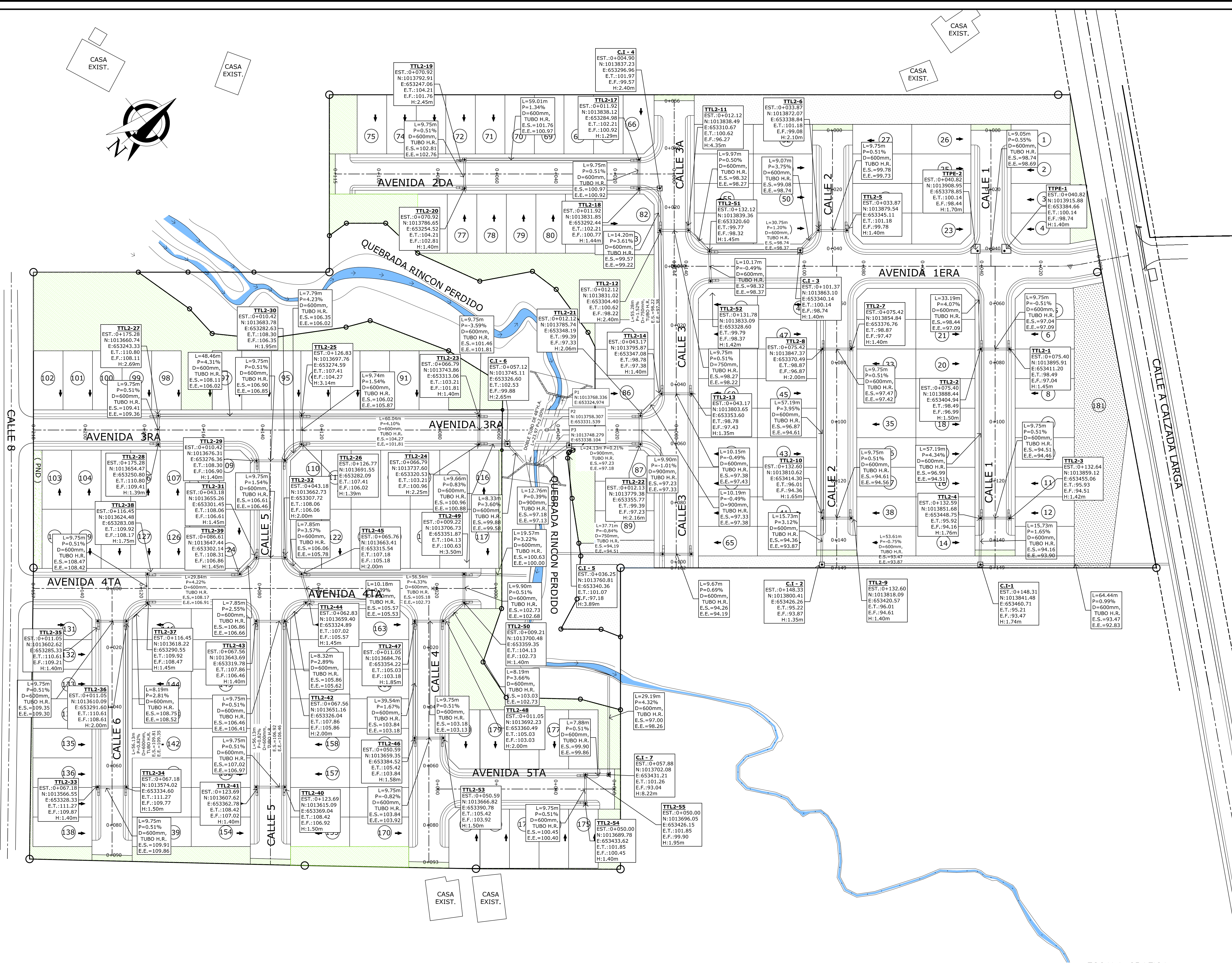
PLANTA DE SISTEMA PLUVIAL ESC. 1 : 600
