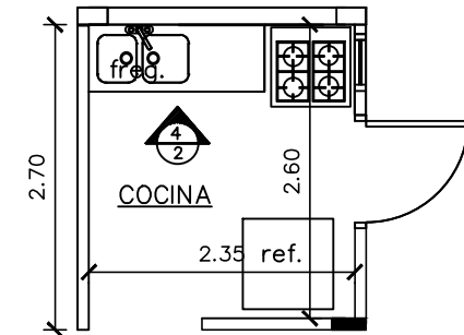
AMPLIACION DE COCINA
