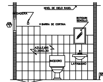
ELEVACION SERV. SANITARIO
