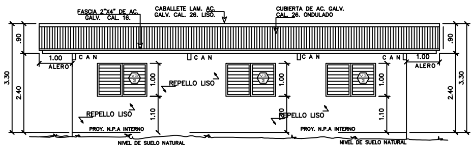
ELEVACION LATERAL IZQUIERDA.
