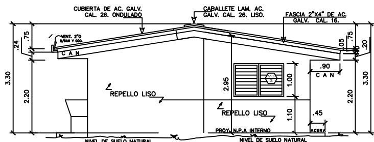
ELEVACION POSTERIOR
