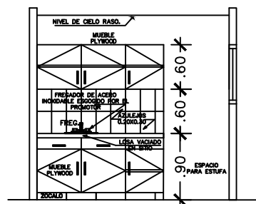
ELEVACION DE COCINA
