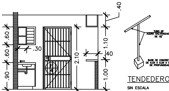
SECCION DE COCINA
