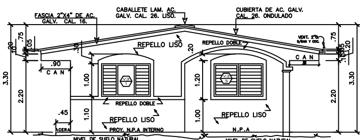
ELEVACION FRONTAL
