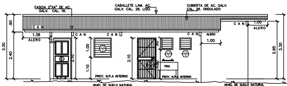
ELEVACION LATERAL DERECHA
