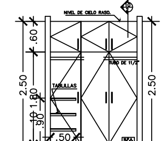
ELEVACION DE CLOSET.
