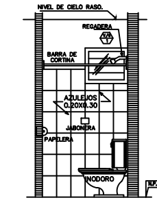
SECCION DE SERV. SANITARIO
