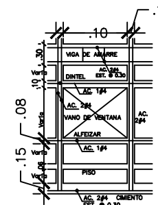
REFUERZO DE VENTANA
