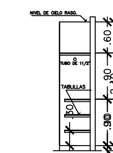
ELEVACION DE CLOSET.
