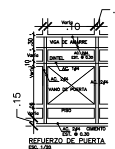
REFUERZO DE PUERTA
