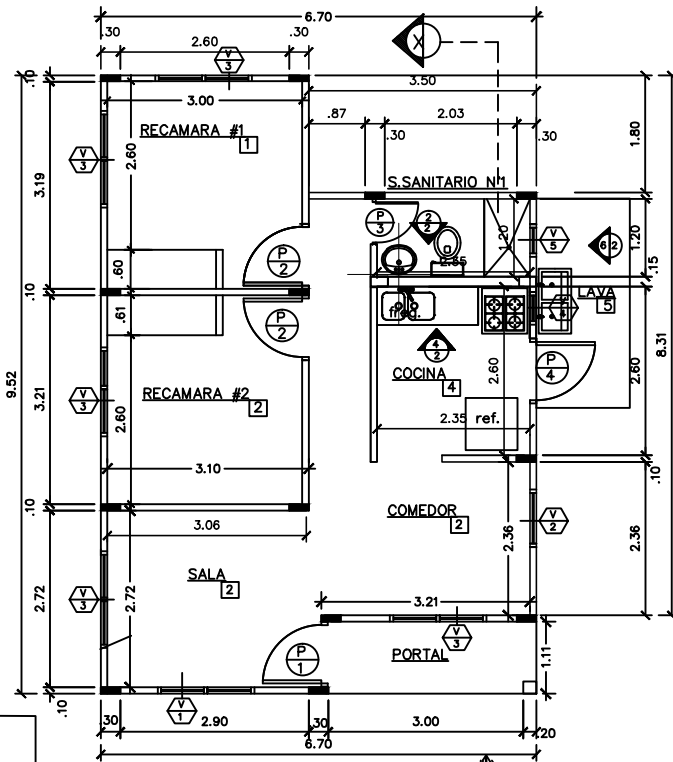
PLANTA ARQUITECTONICA MODELO "C" 2 REC. 54.00 M 2
