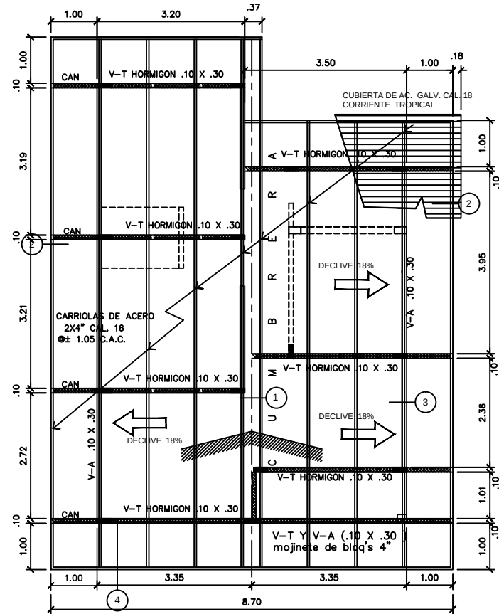
ESTRUCTURA DEL TECHO AREA DE CUBIERTA= 92.80 M 2
