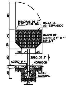
ELEVACION LAT. DE TINAQUERA ESC. 1 : 20
