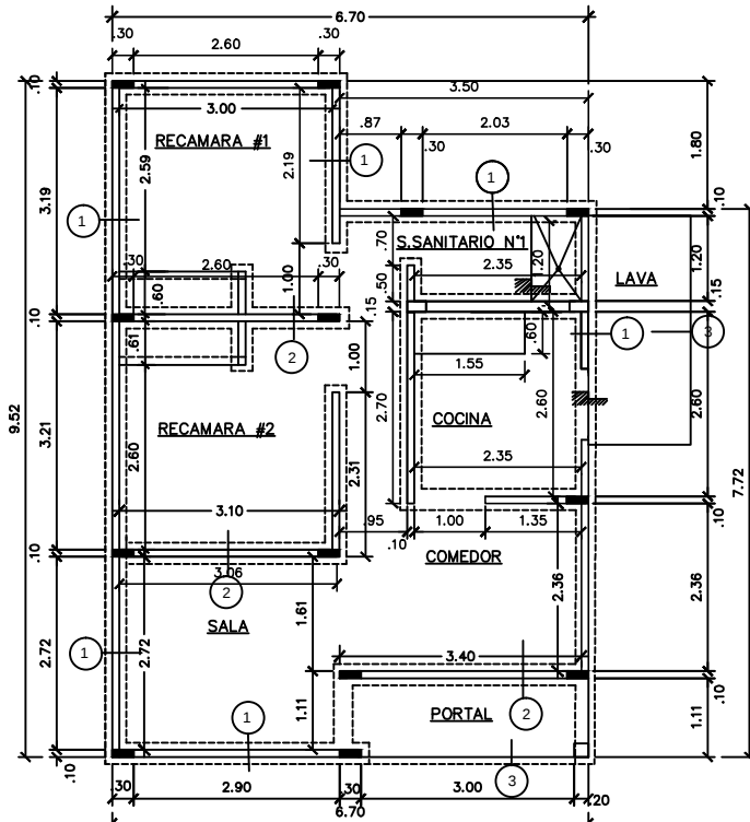
PLANTA DE CIMIENTOS COORDINAR MEDIDAS CON LA PLANTA ARQUITECTONICA
