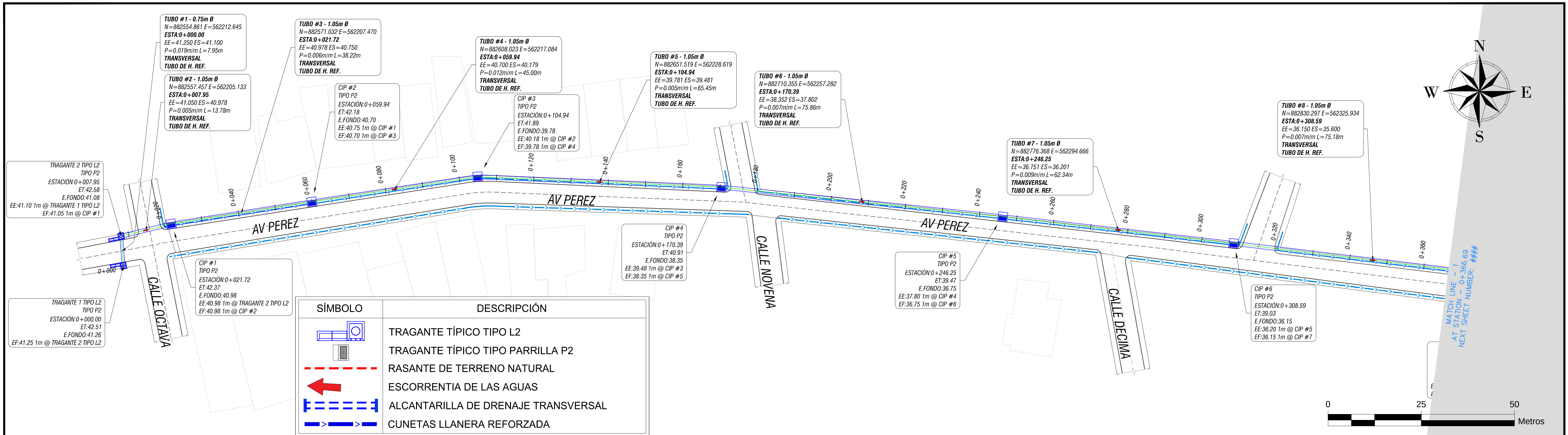
PLANTA - PERFIL 0+000.00 - 0+368.00
