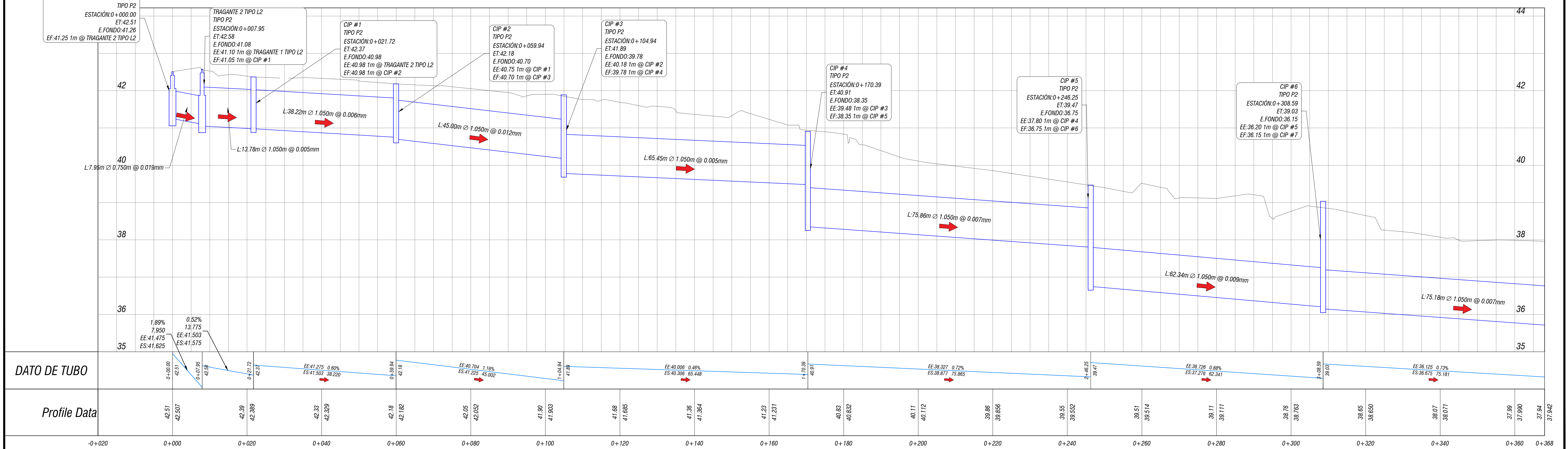
PLANTA - PERFIL 0+000.00 - 0+368.00
