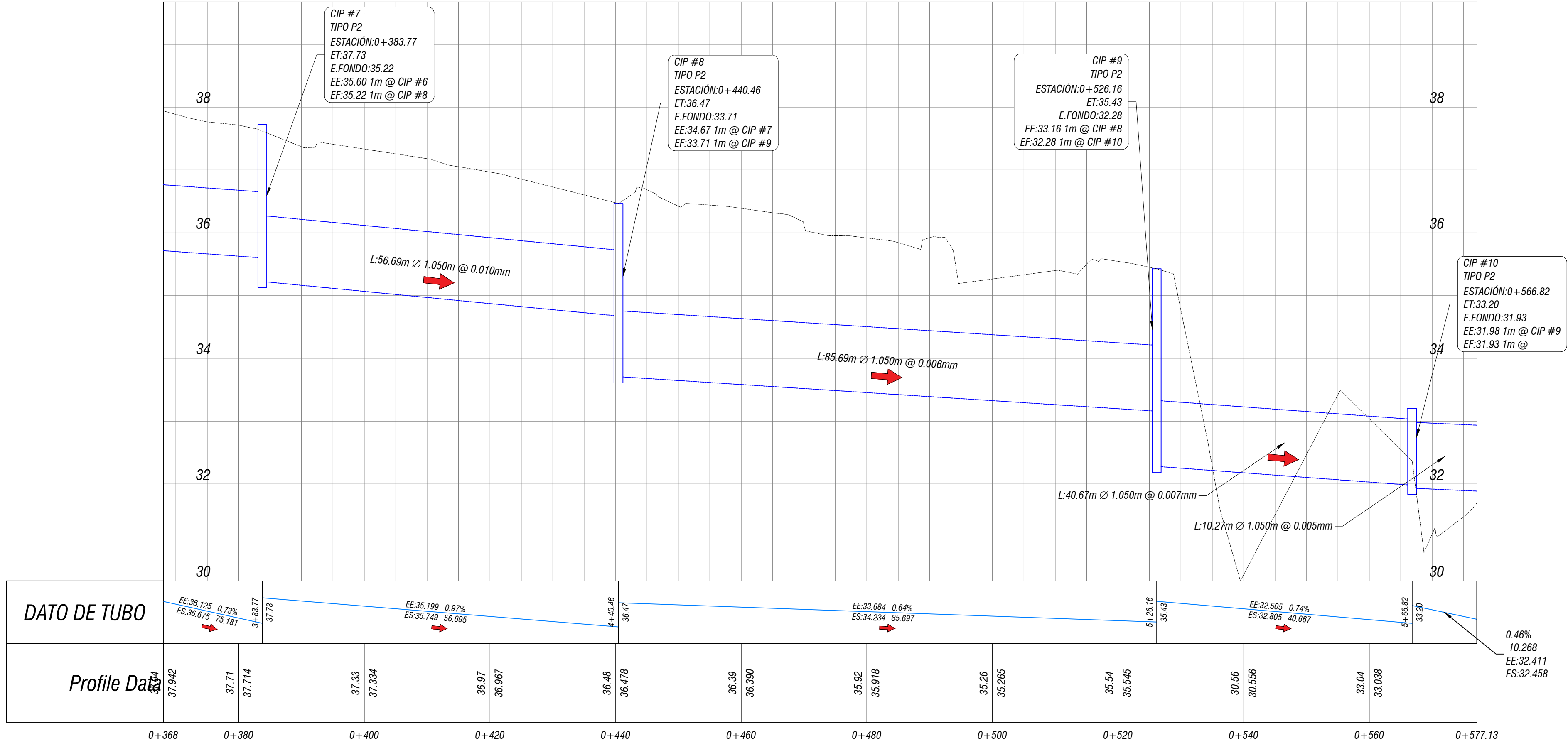
PLANTA - PERFIL 0+368.00 - 0+577.13
