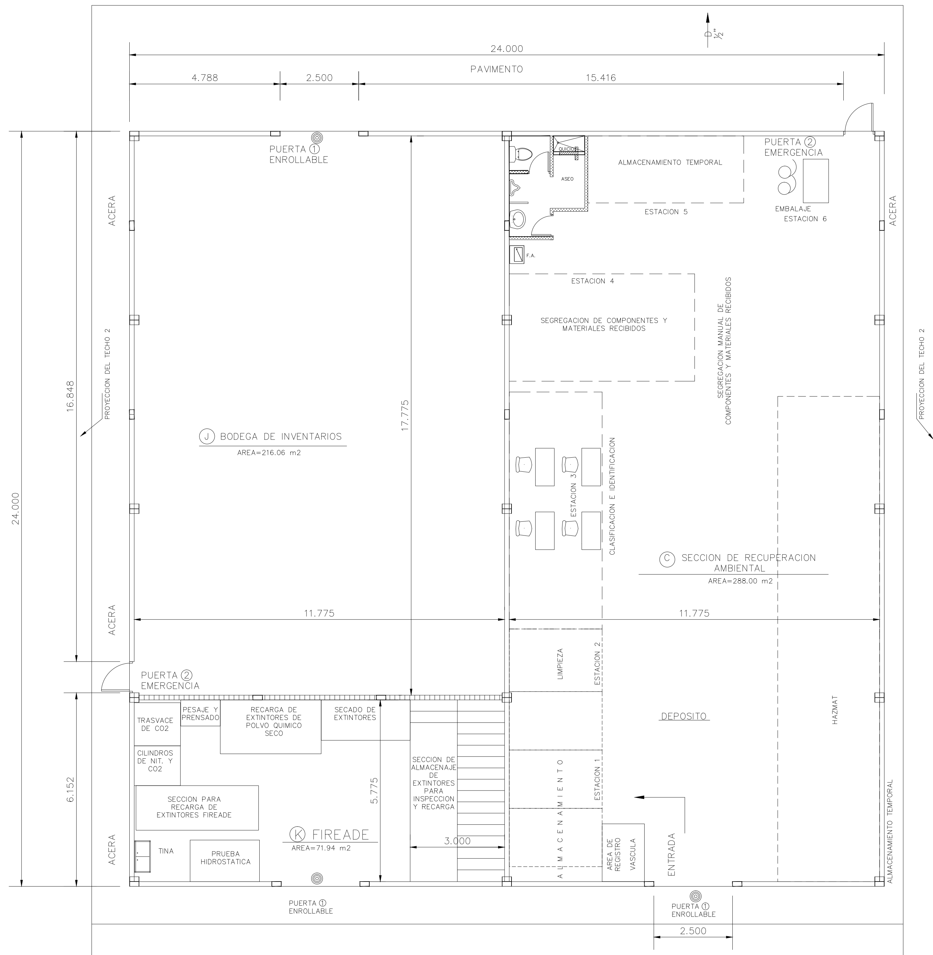
PLANTA DE GALERA MULTIUSO
