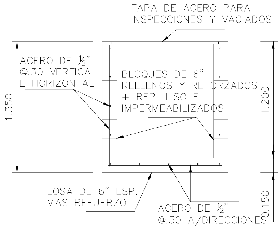
SECCION ESC: 1:40
