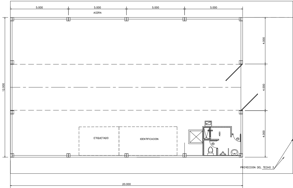
GALERA E EQUIPAMIENTO PARA OPERACIONES INTERNAS AREA CERRADA = 240.00 m2 BSC. 1 : 75
