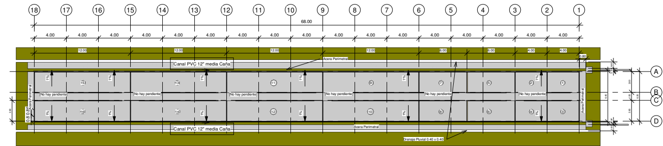
Planta Piso Acotada
