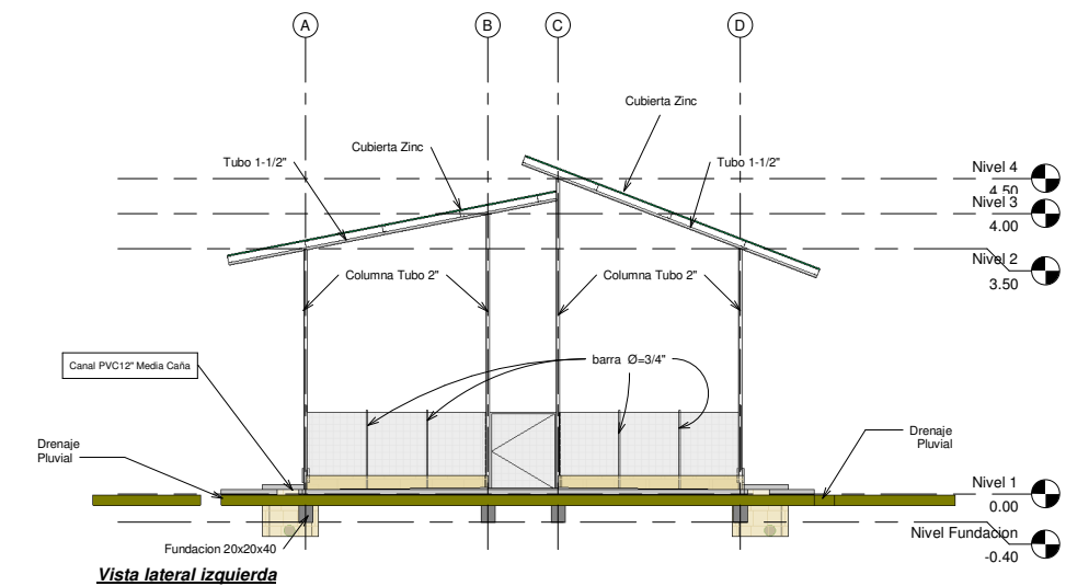
5 Oeste 1 : 50
