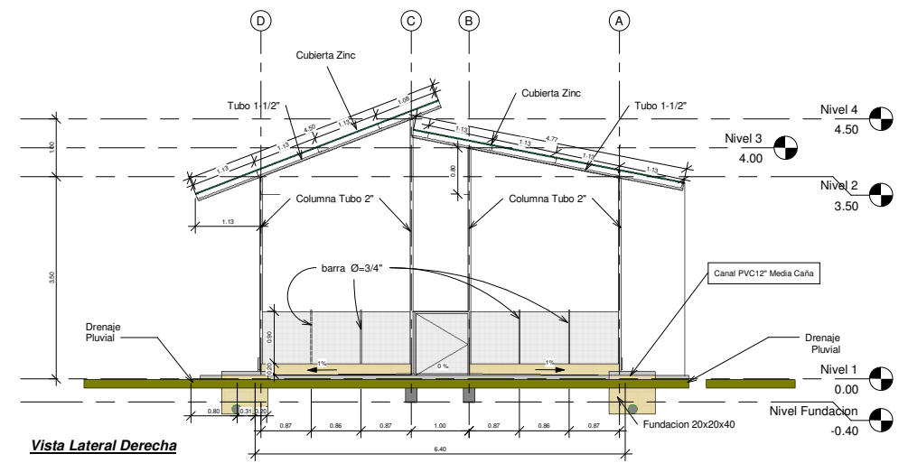
3 Este 1 : 50
