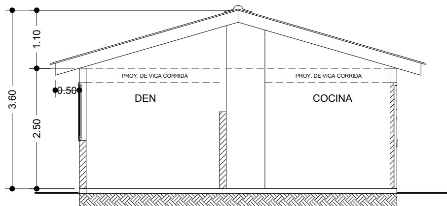
CORTE TRANSVERSAL B - B
