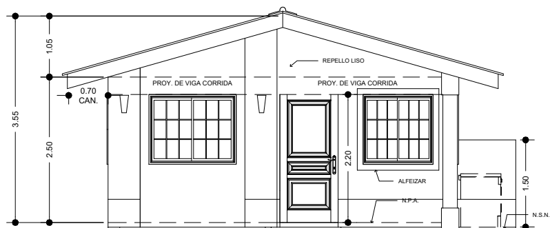
ELEVACION FRONTAL
