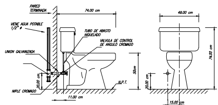
DET. DE CONEXIÓN DE INODORO SIN ESCALA
