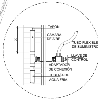
LLAVE DE PASO EN ARTEFACTO SANITARIO ESCALA: 1 : 100
