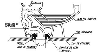
DIAGRAMA DE LA TAZA SOBRE LA BRIDA SIN ESCALA
