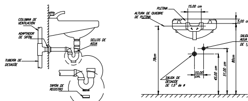
INSTALACIÓN DE LAVAMANOS SIN ESCALA
