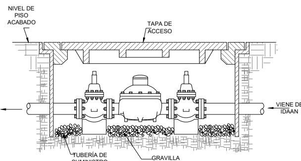
DETALLE DE INSTALACIÓN INSTALACIÓN DE MEDIDOR OPCIONAL PARA EL PROPIETARIO SIN ESCALA
