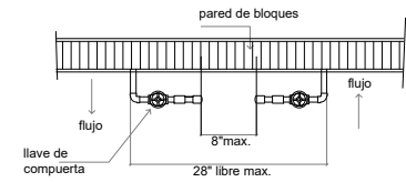
PLANTA DE MEDIDORES SIN ESCALA
