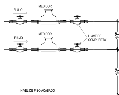
ELEVACIÓN TÍPICA DE CONEXIÓN DE AGUA POTABLE SIN ESCALA
