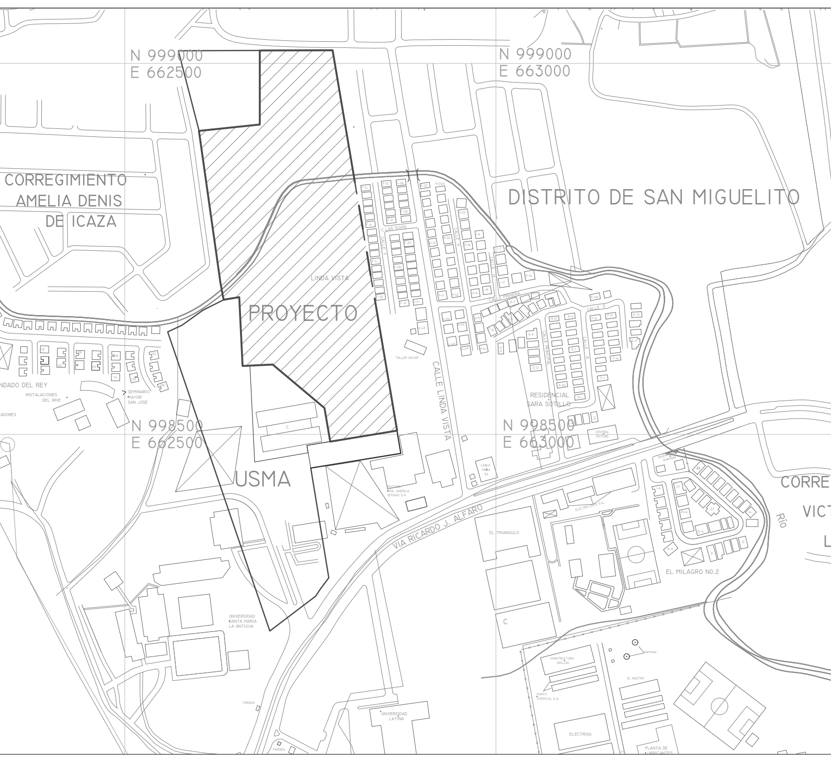
1 UBICACION REGIONAL ESC.: 1/20,000
