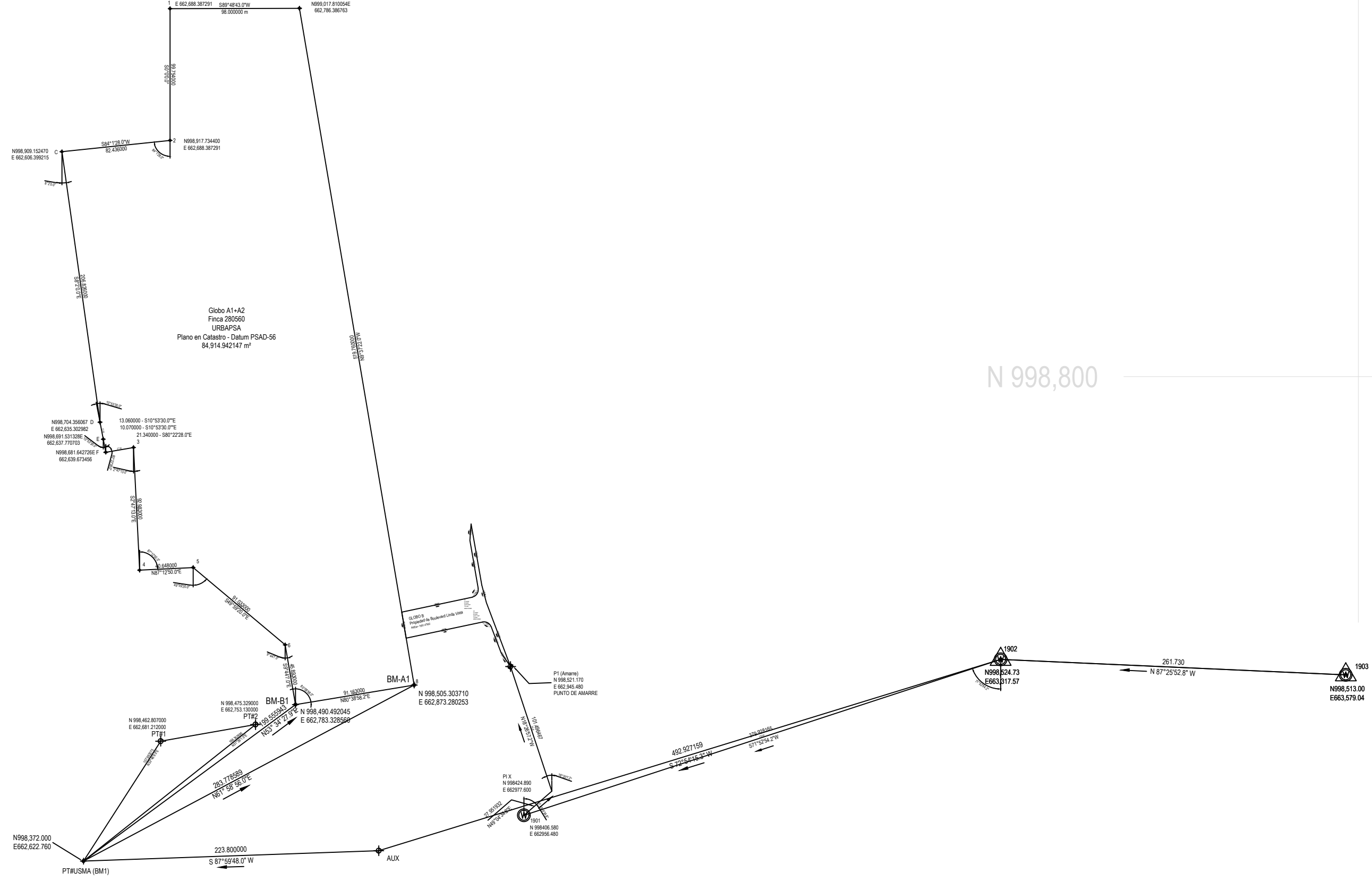
2 DETALLE DE AMARRE ESC.: 1/3,000
