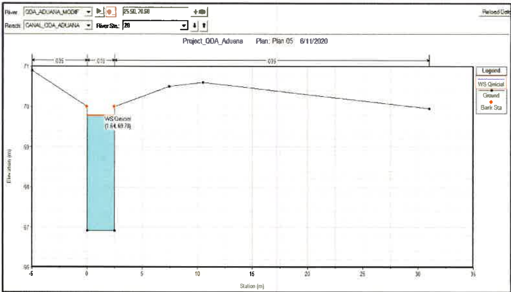
Figura A.5.1.2. Secciones transversales usadas para alimentar el programa HEC-RAS. Estación 20 del cauce de la quebrada Sin Nombre, aguas arriba.
