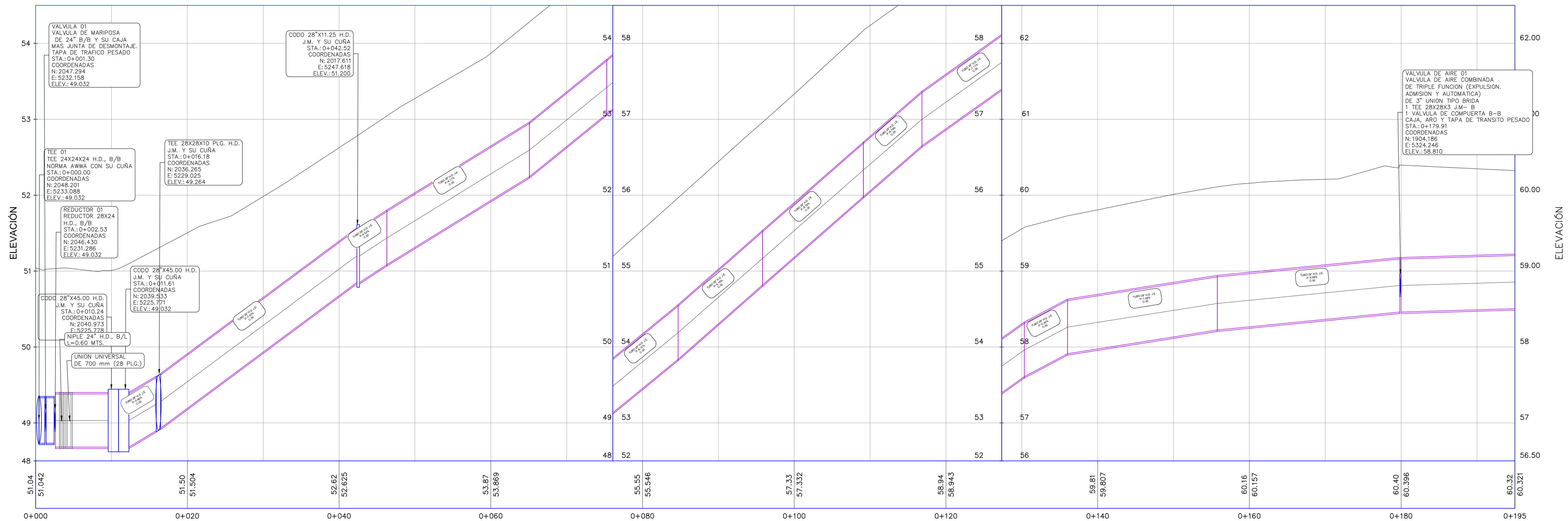
Tubería_28plg PROFILE
