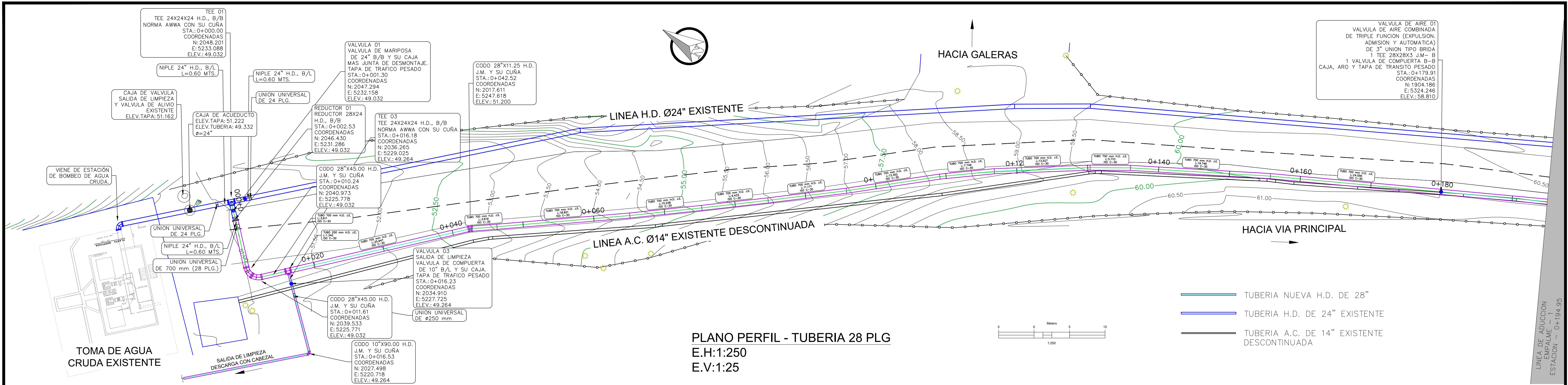
Tubería_28plg PROFILE
