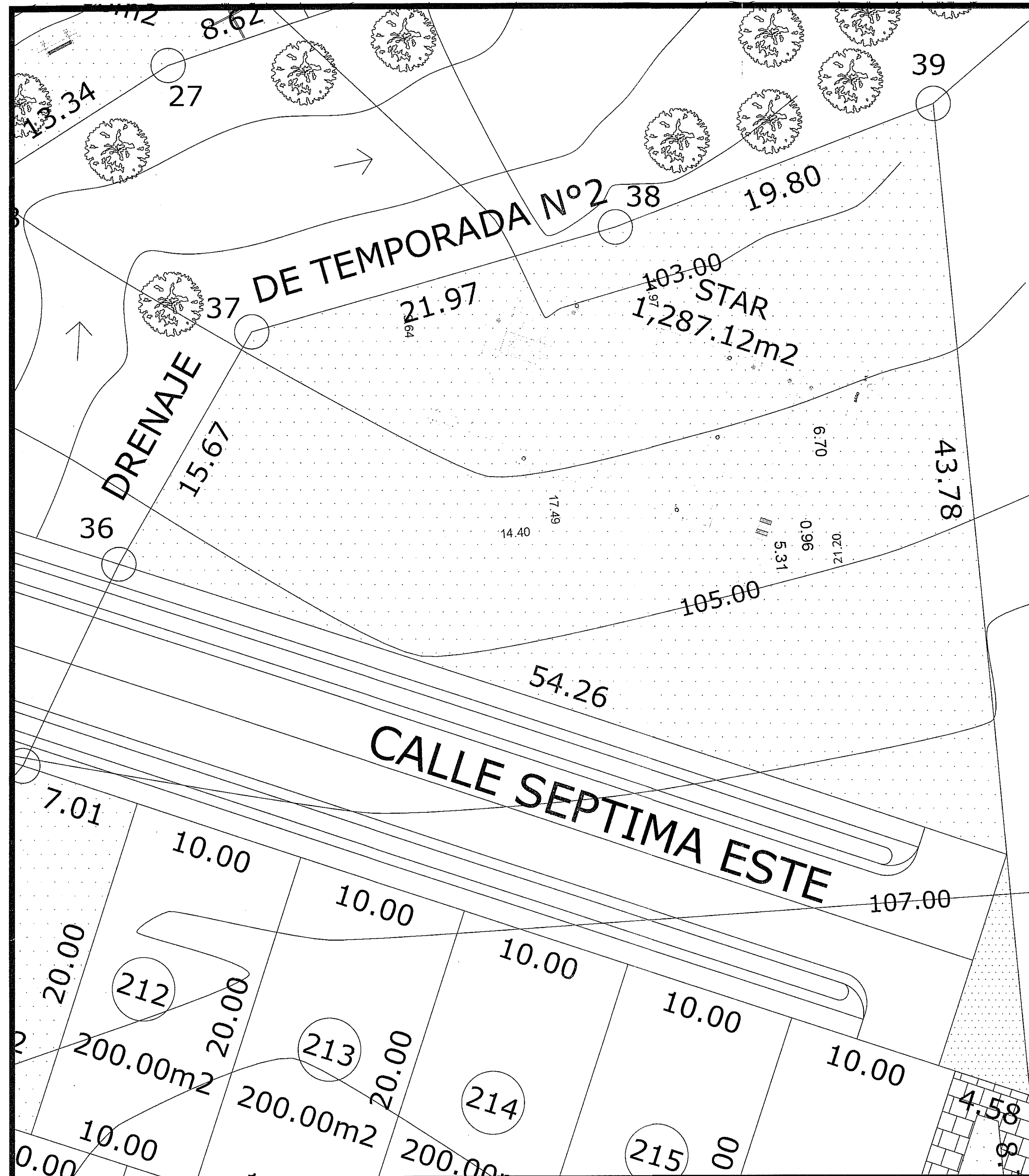
P LANTA DE RETIROS SISTEMA DE TRATAMIENTO DE AGUAS RESIDUALES
