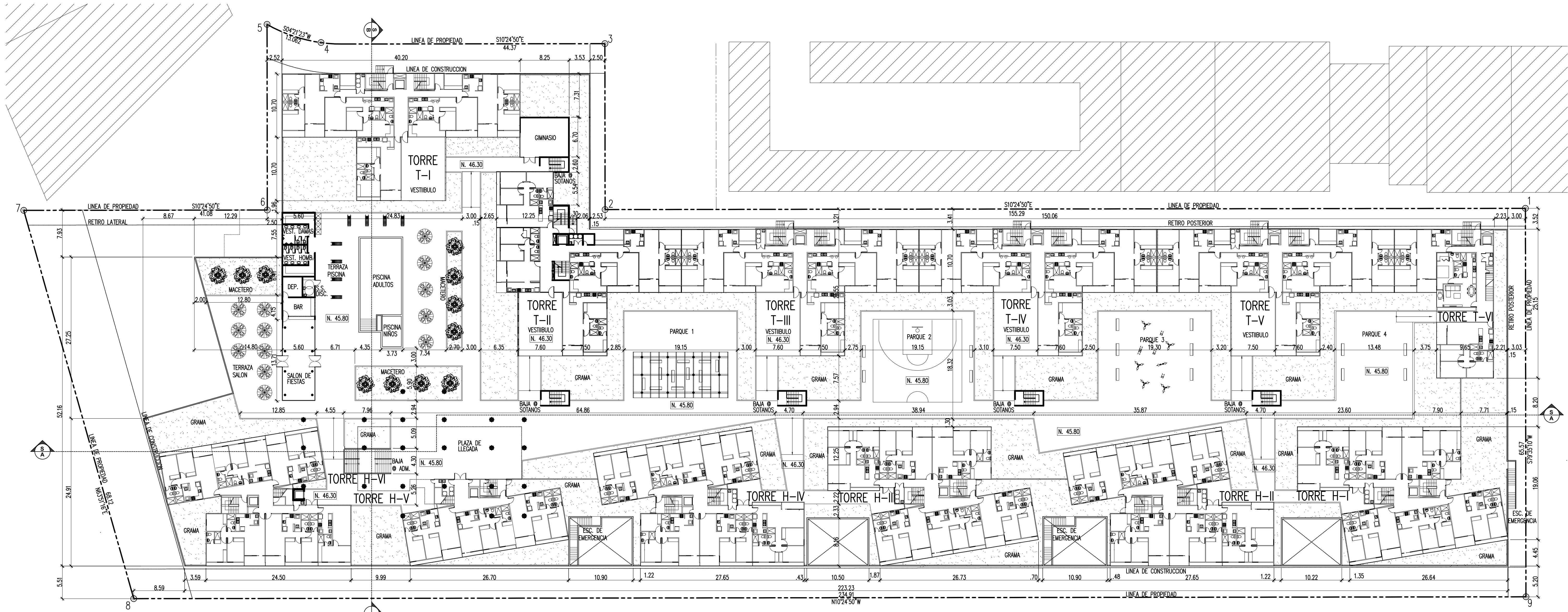
PLANTA ARQUITECTONICA DEL CONJUNTO (NIVEL 100)
