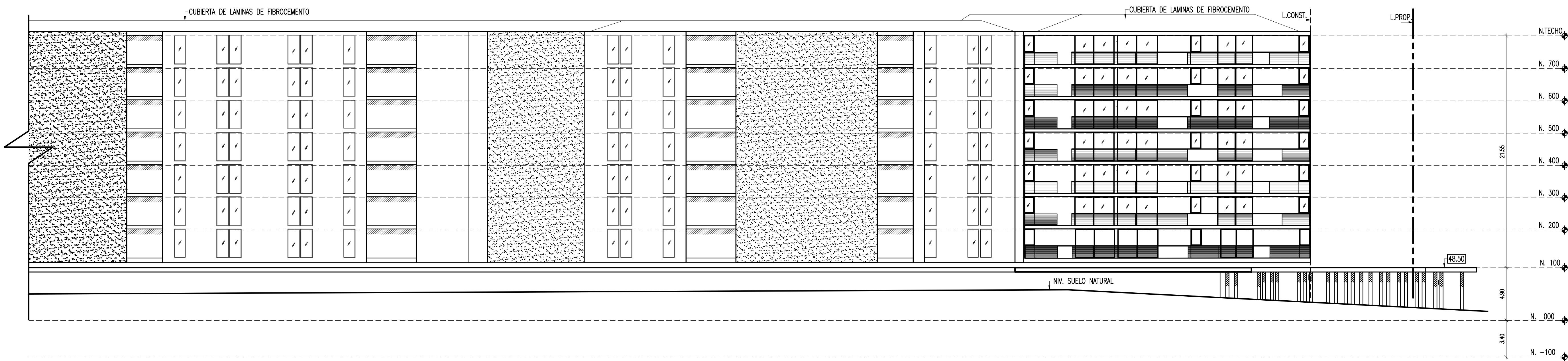
ELEVACION OESTE - PARCIAL DER.
