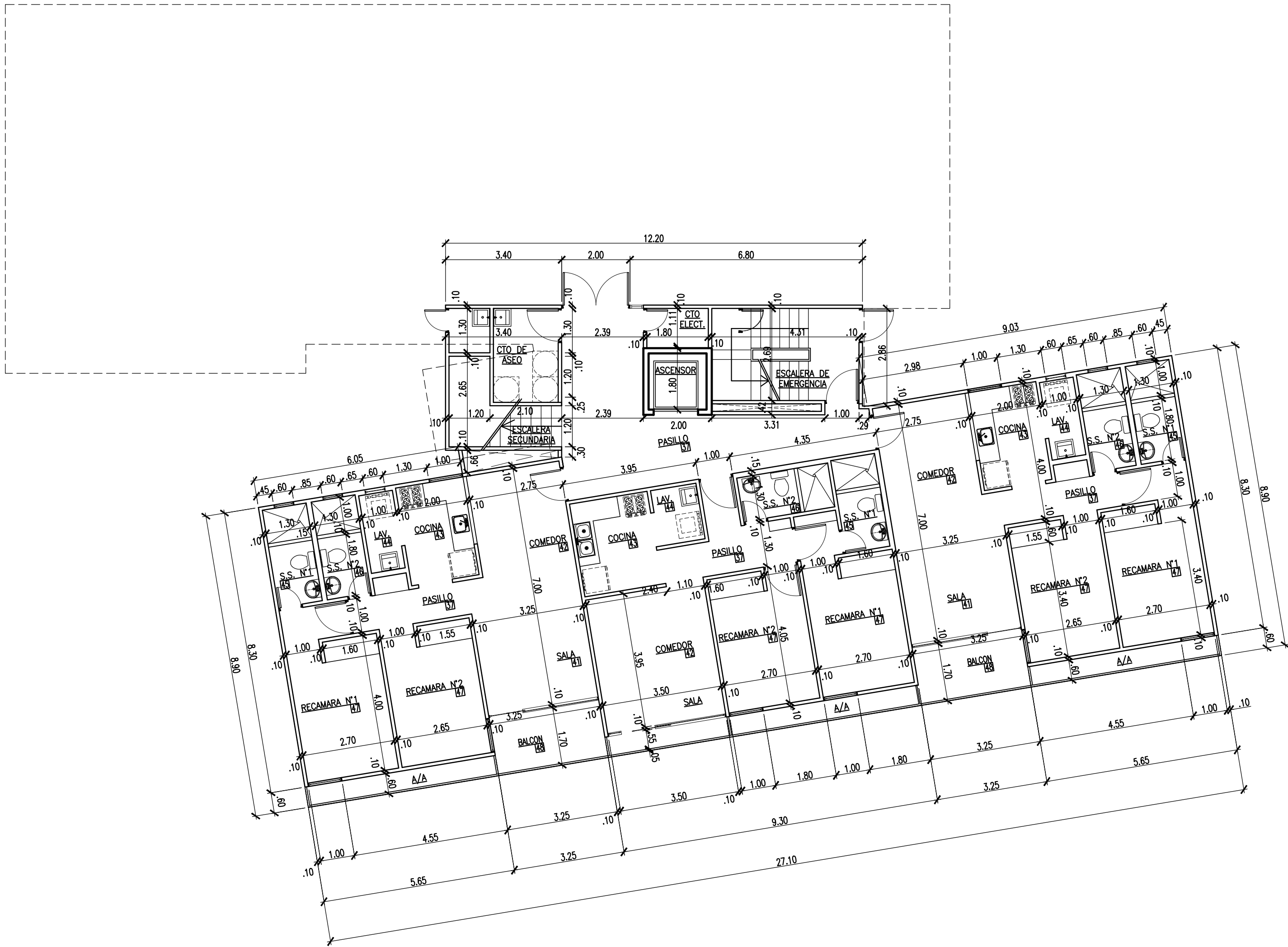
PLANTA ARQUITECTONICA NIV 100 - TORRE TIPO HB
