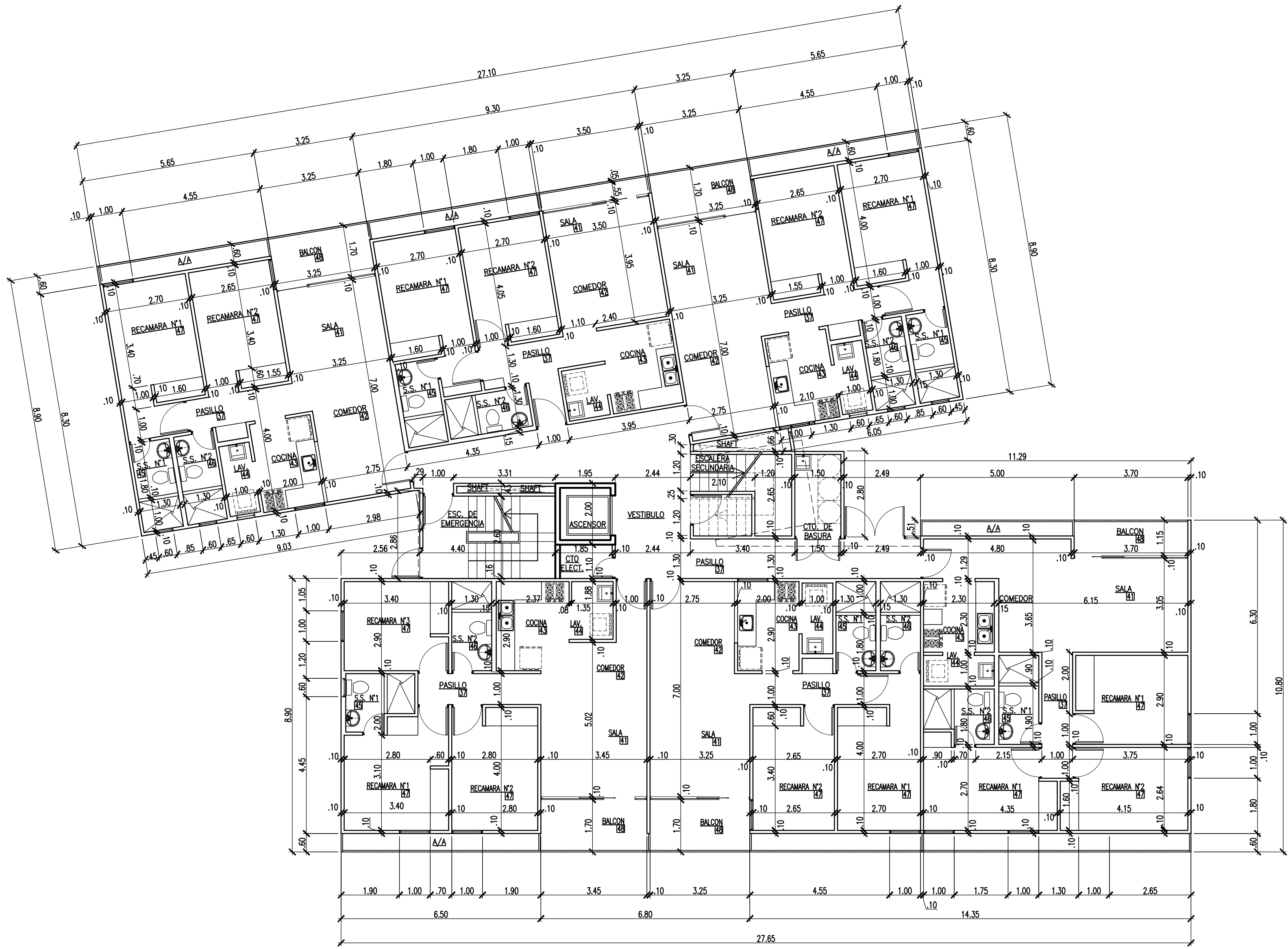
PLANTA ARQUITECTONICA NIV 100 - TORRE TIPO HA
