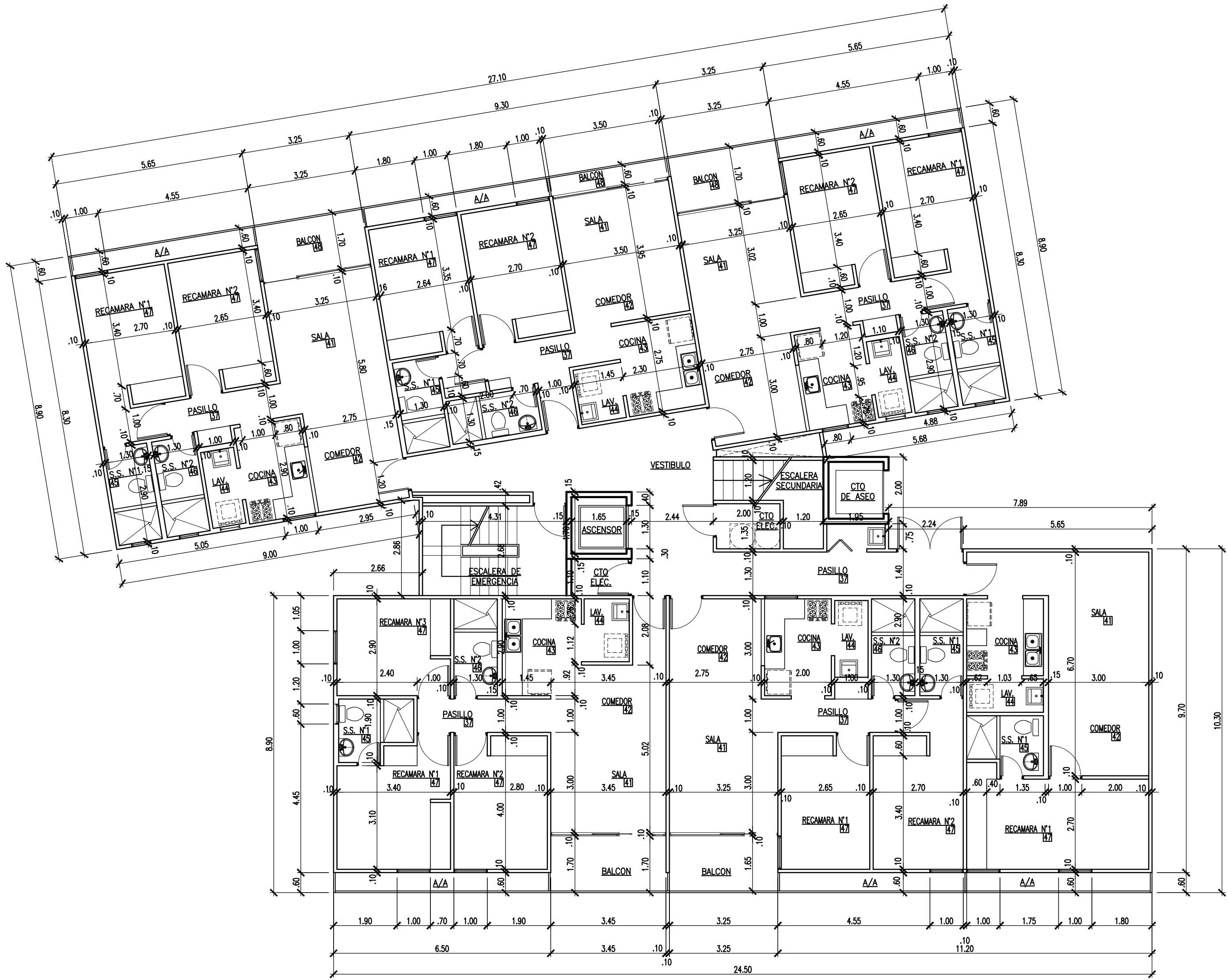
PLANTA ARQUITECTONICA NIV 100 - TORRE TIPO HC
