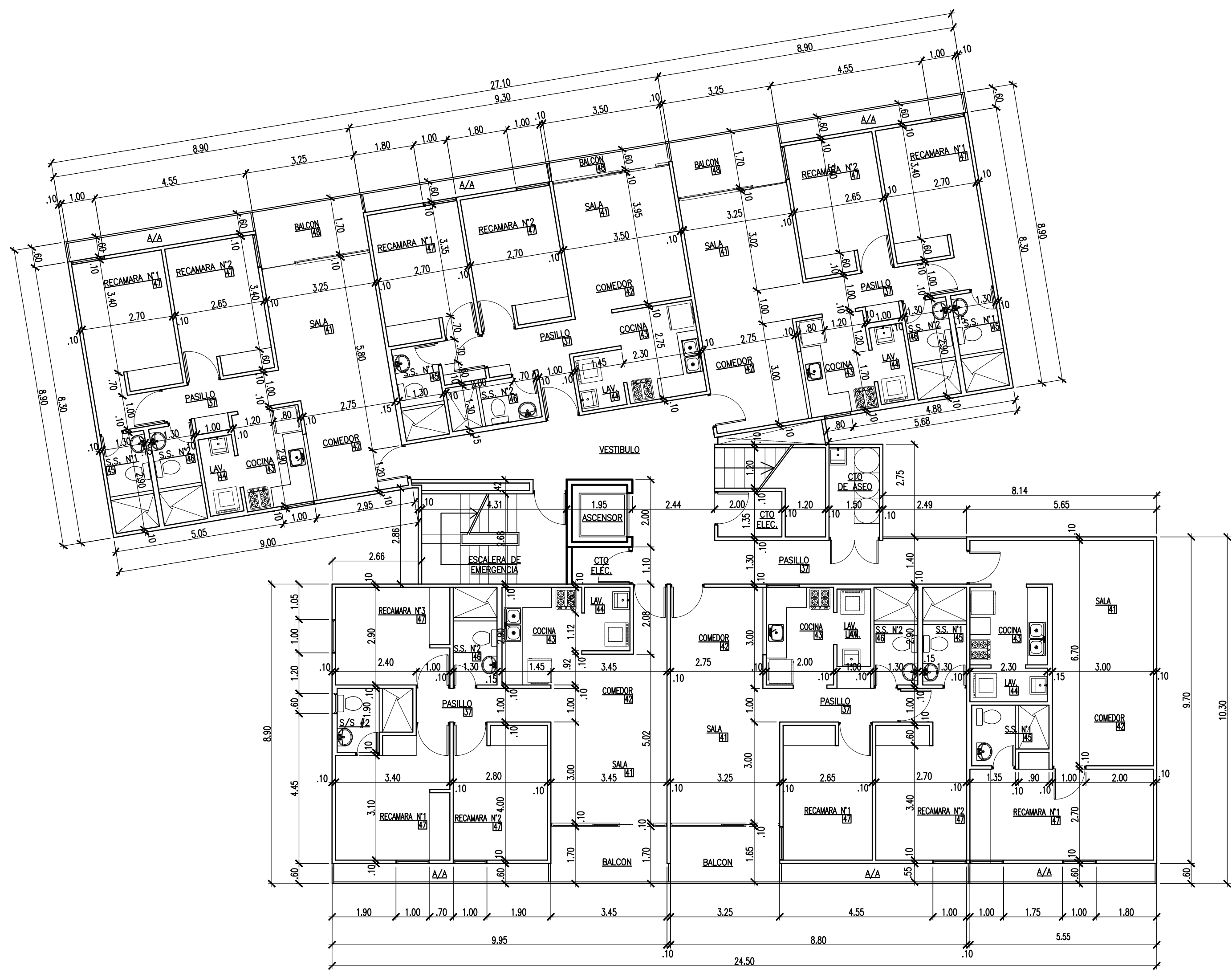
PLANTA ARQUITECTONICA NIVEL 200 @ 700 - TORRE TIPO HC
