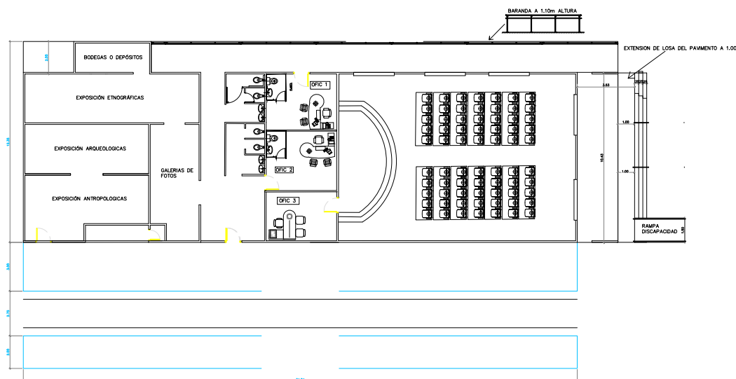
PLANTA ARQUITECTONICA (NUEVA)
