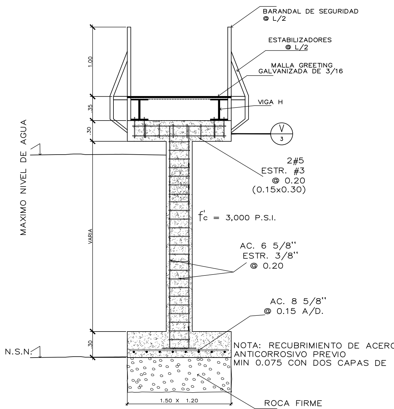
SECCION DE ATRACADERO ESCALA 1/33
