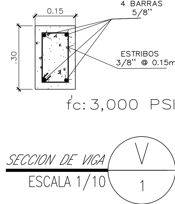
SECCION VIGA H ESCALA 1/10
