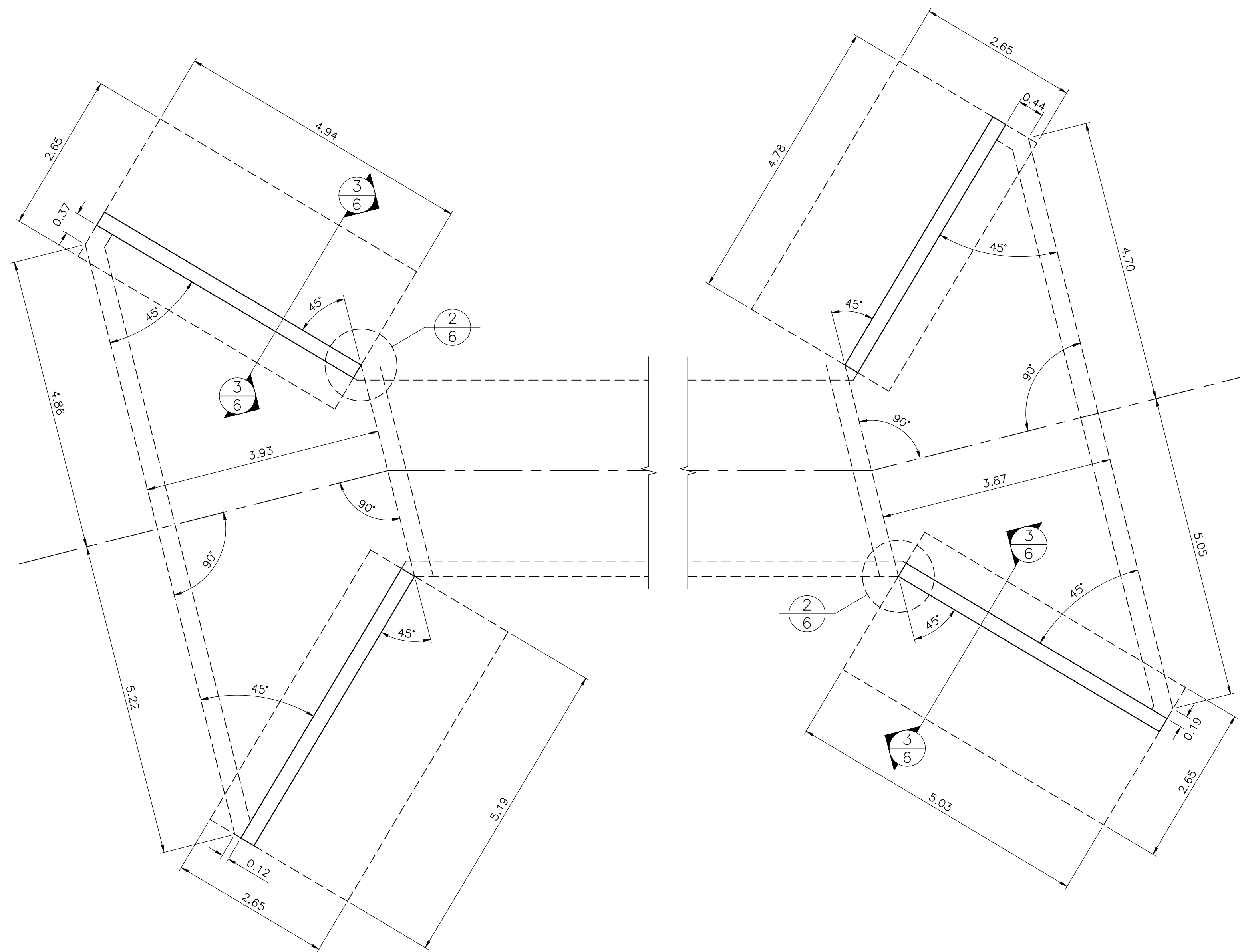
1 PLANTA DE DERRAMADERO DE SALIDA ESCALA 1:50
