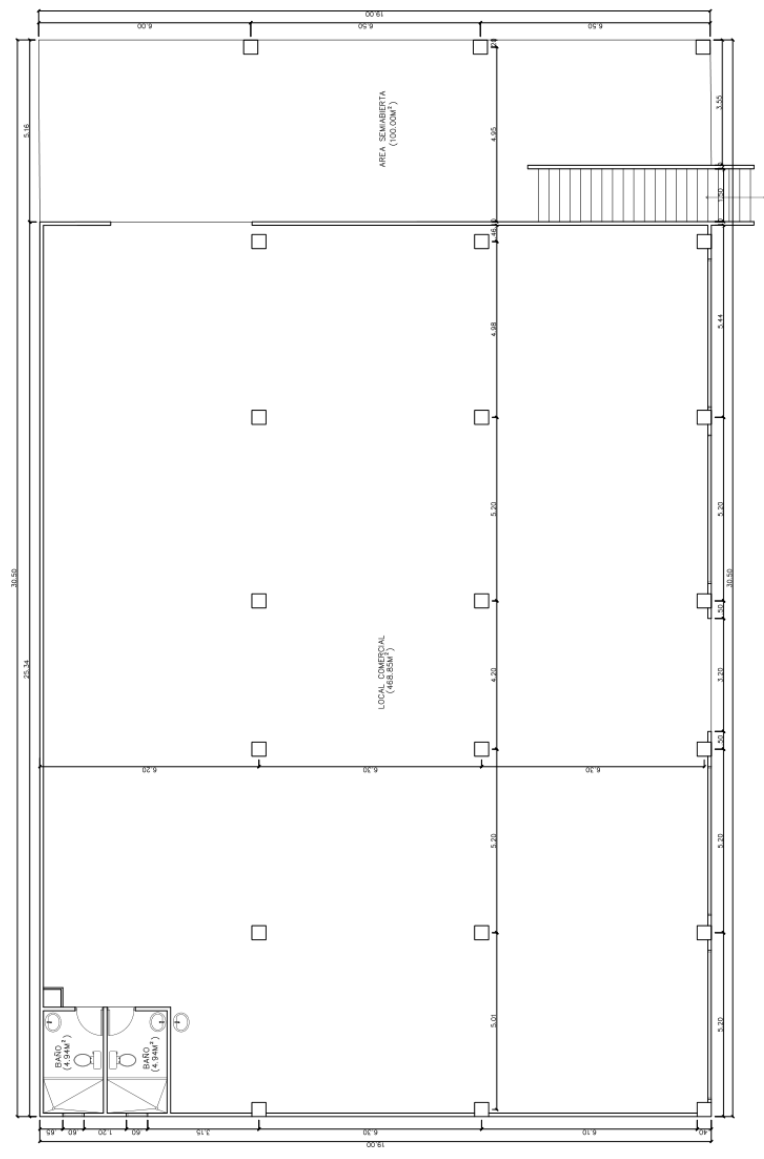
Figura 5. Planta arquitectónica baja (Fuente: Planos del proyecto)
