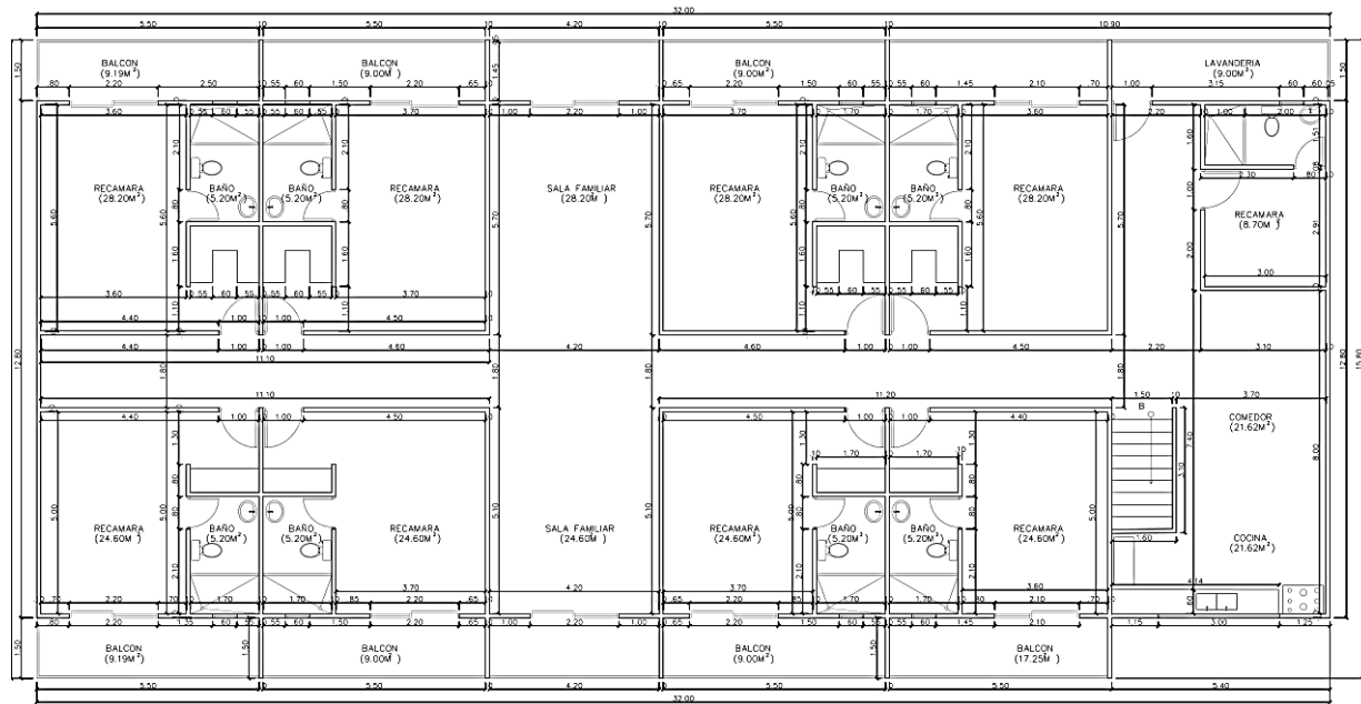
Figura 6. Planta arquitectónica alta (Fuente: Planos del proyecto)
