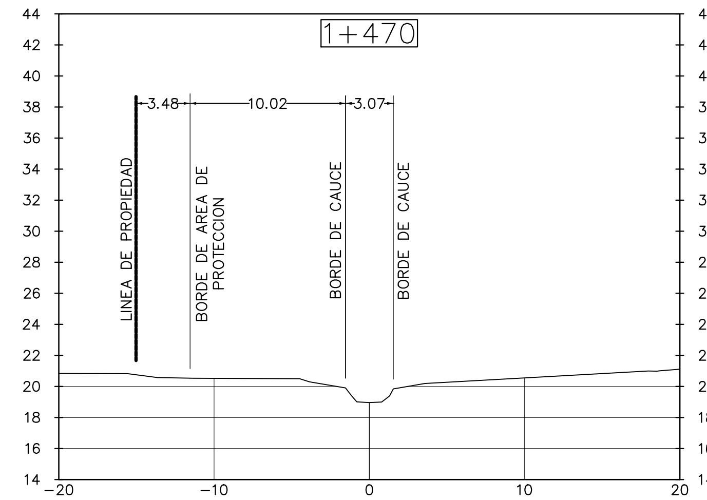
SECCIONES QUEBRADA CAÑA BRAVA ESC: 1:250
