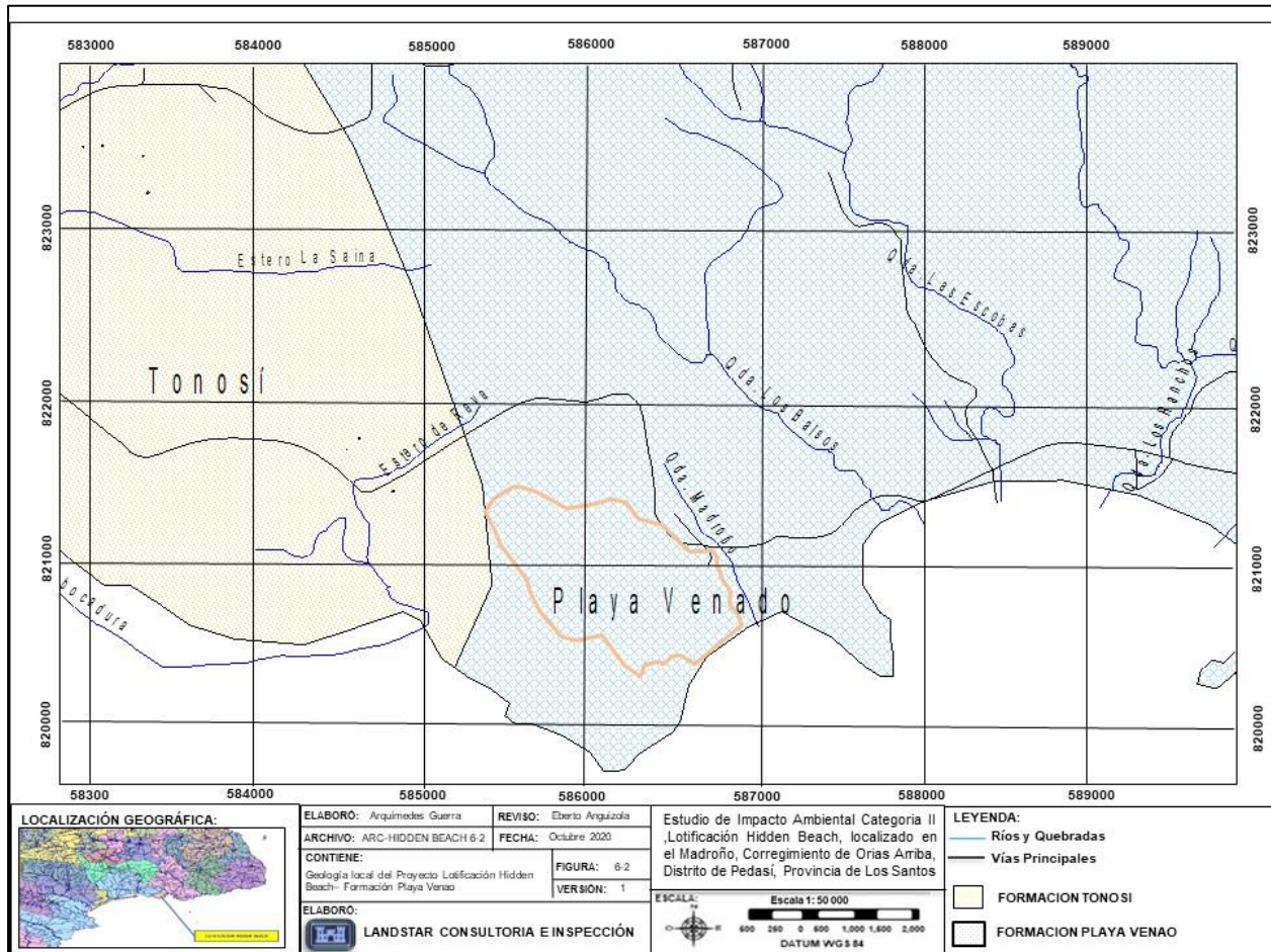
Mapa N°6-2: Unidades Geológicas Locales Escala 1:50 000.LANDASTAR 2020
