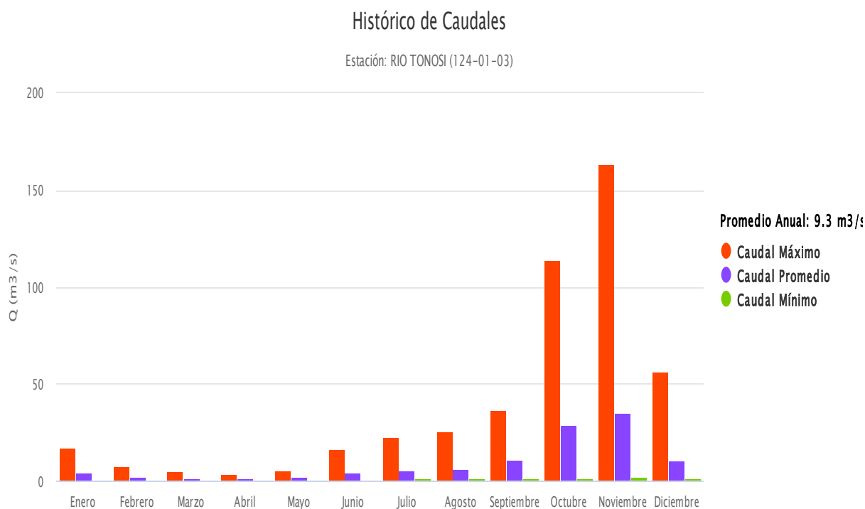
Gráfico N°6-9: Caudales en (m³/s) de la estación utilizada para el traslado de caudales 124-01-03 ubicada en el puente del río Tonosi (1999-2019)
