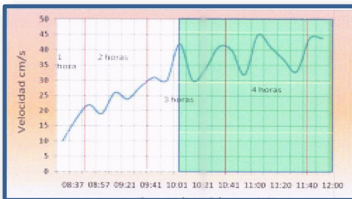
Gráfico N°6-10 Velocidad de Corriente vs. Tiempo Estado Vaciente en Sicigia, Costas de Azuero. Información Suministrada por LANDSTAR CONSULTORIA & INSPECCION -2020
