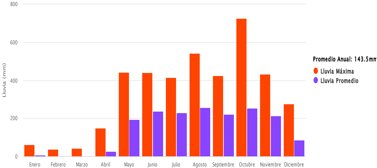
Gráfico N°6-6: Precipitación Máxima y Promedio de la estación 126-015 (1974-2019). Elevación 8.0 m nmm.
