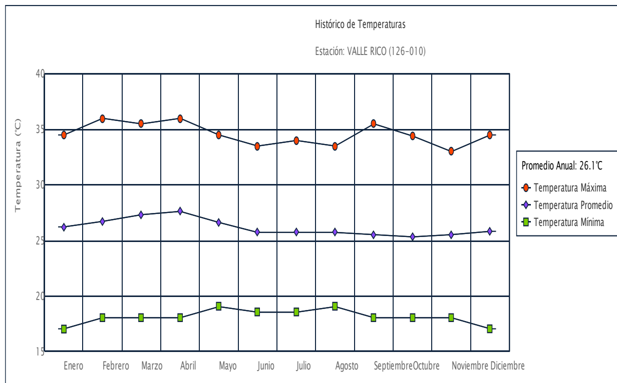
Gráfico N°6-1: Temperaturas Máximas, Mínimas y Promedio de la Estación 126-010- (1972-2019). Información ETESA-2020
