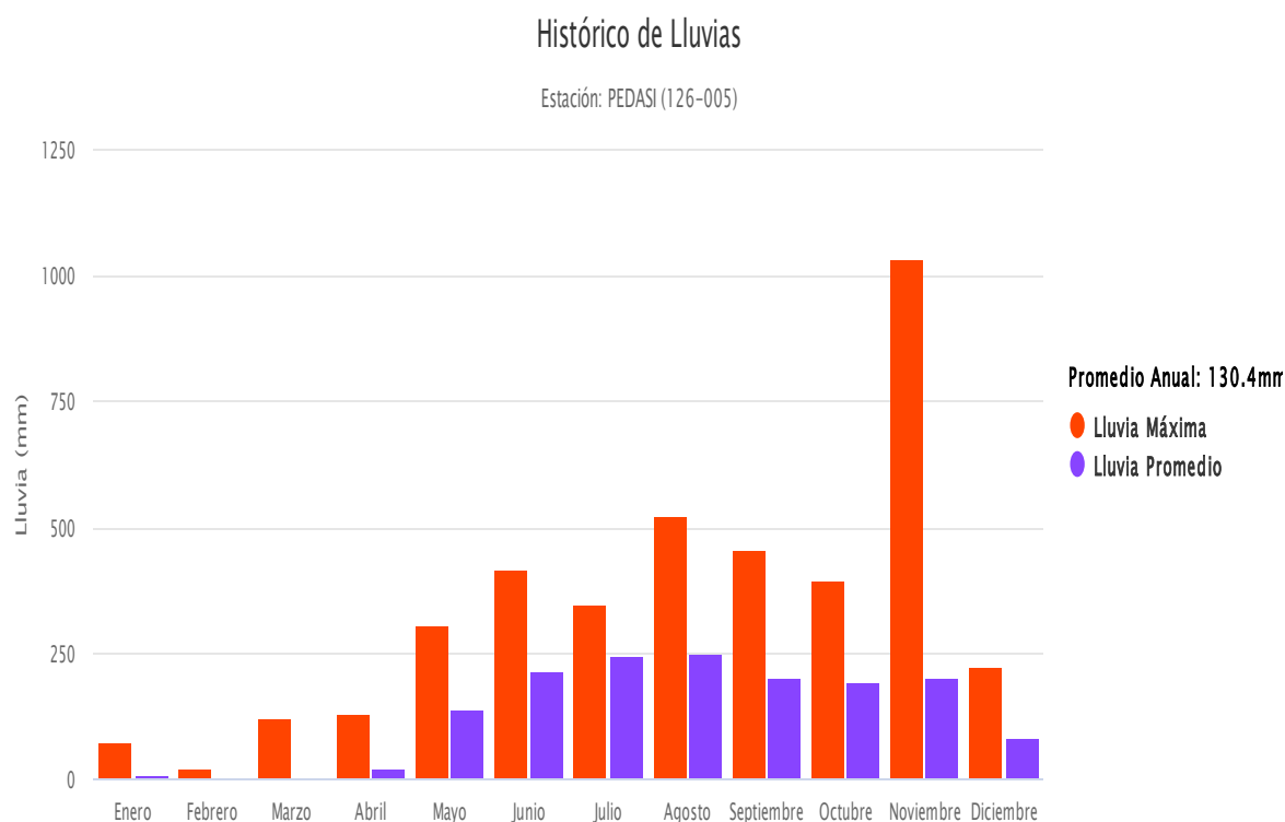
Gráfico N°6-8: Precipitación Máxima y Promedio de la estación PEDASI 126-005 periodo (1967-2019). Elevación 47 msnm
