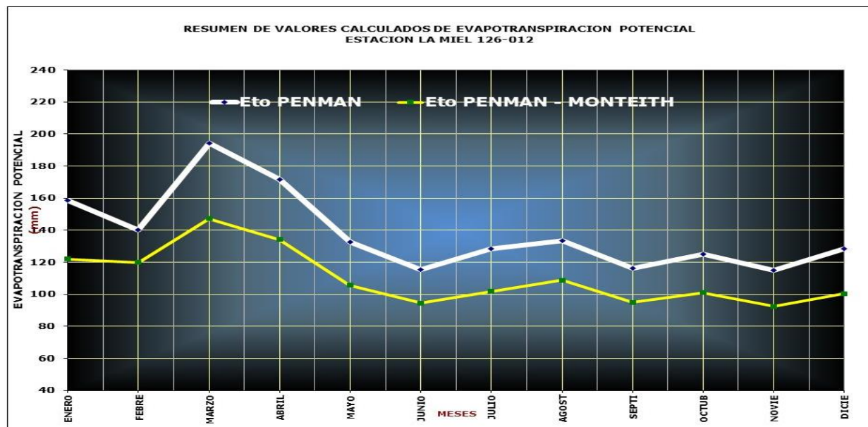
Gráfico N°6-4: Evapotranspiración Potencial Calculada para Microcuenca de la Quebrada Madroño. Se utilizo el Eto PENMAN-MONTEITH -LA MIEL 126-012
