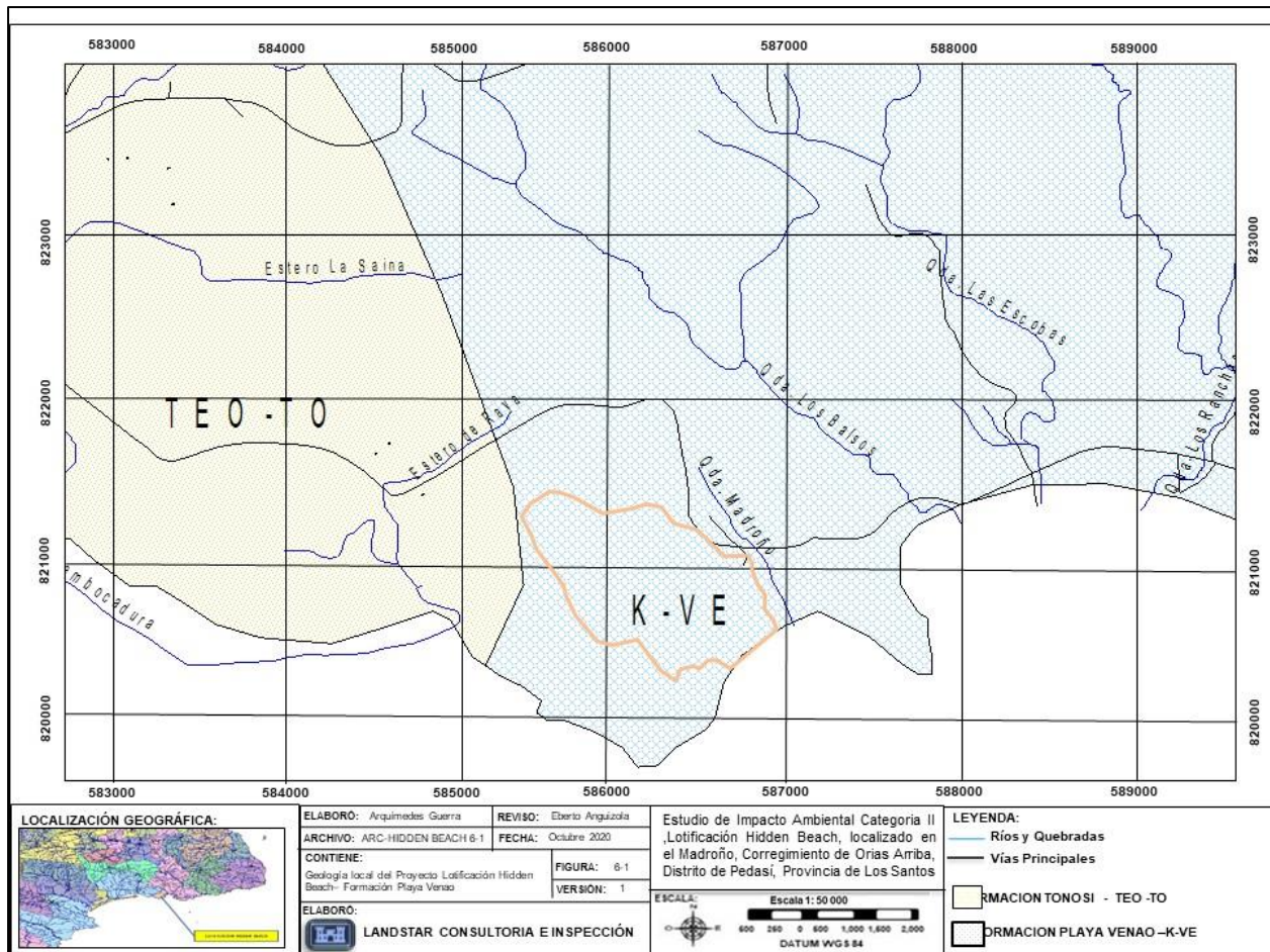
Mapa N°6-1: Unidades Geológicas Regionales Escala 1:50 000.LANDASTAR 2020
