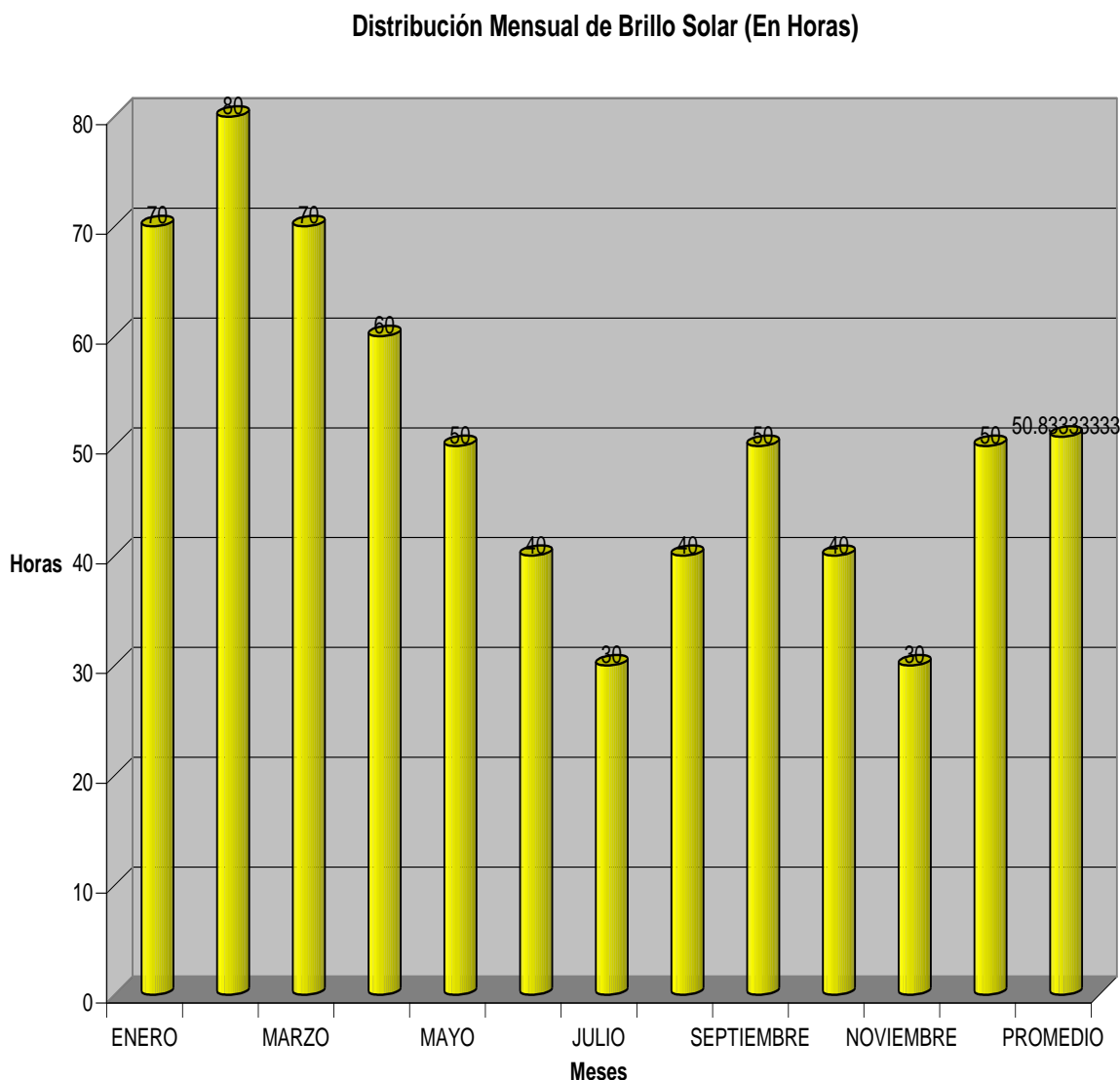
Gráfico N°6-5: Porcentaje de Brillo Solar. Subcuenca Quebrada Madroño (2013-2019). Valores calculados de la estación TONOSI2 124-004. Información ETESA Calculada 2019
