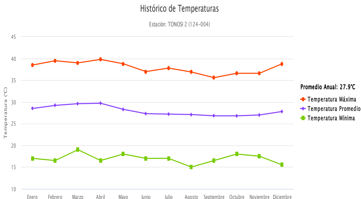
Gráfico N°6-2: Temperaturas Máximas, Mínimas y Promedio de la Estación 124-004- (1972-2019). Información ETESA-2020
