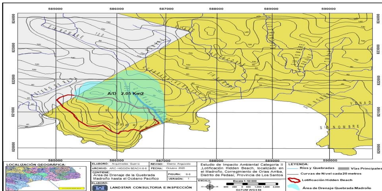
Mapa N°6-6: Área de Drenaje de la Quebrada Madroño. Escala 1:50 000. Elaborado por Landstar Consultoría & Inspección 2020.
