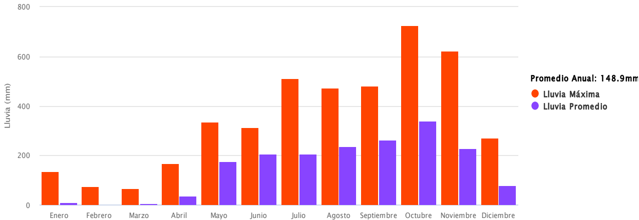
Gráfico N°6-7: Precipitación Máxima y Promedio de la estación La Miel 126-012 (1972-2019). Elevación 220 m msnm.
