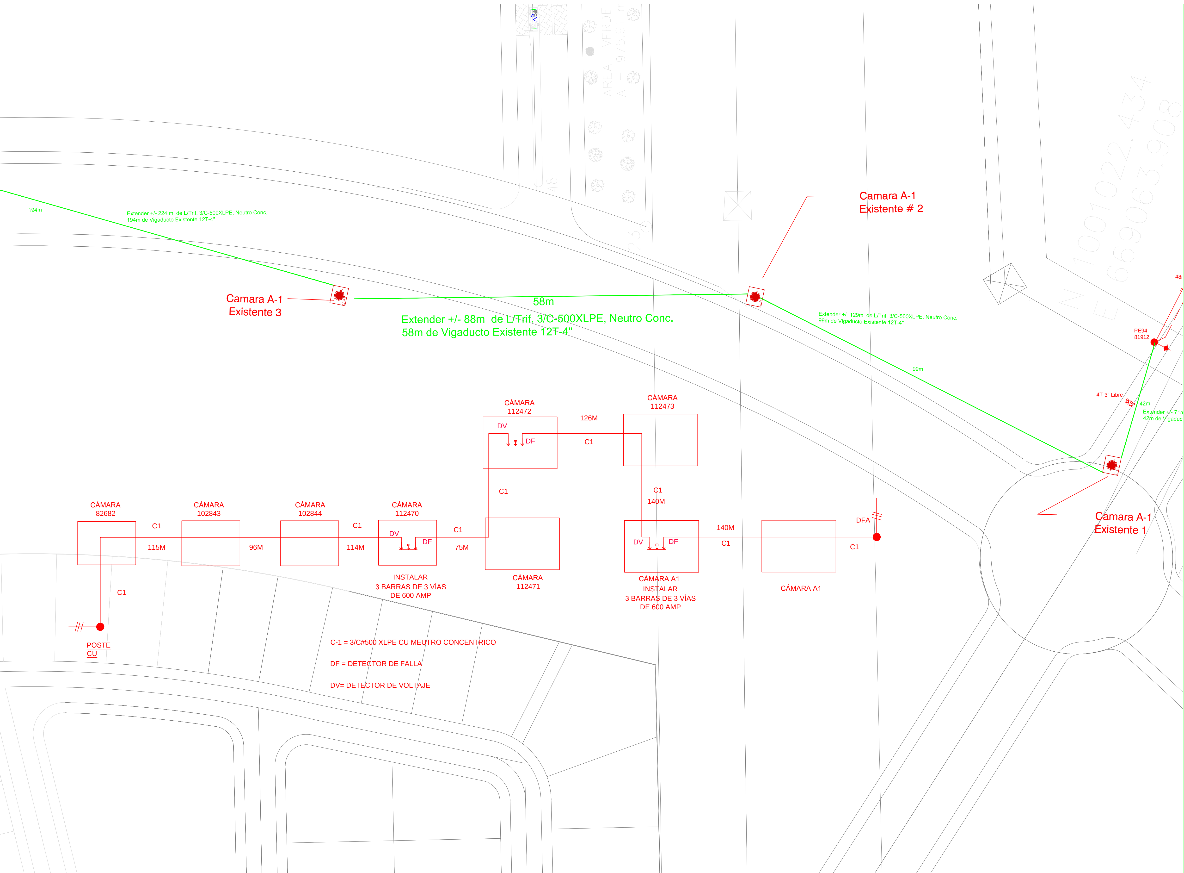
PLANTA ESC: 1/750
